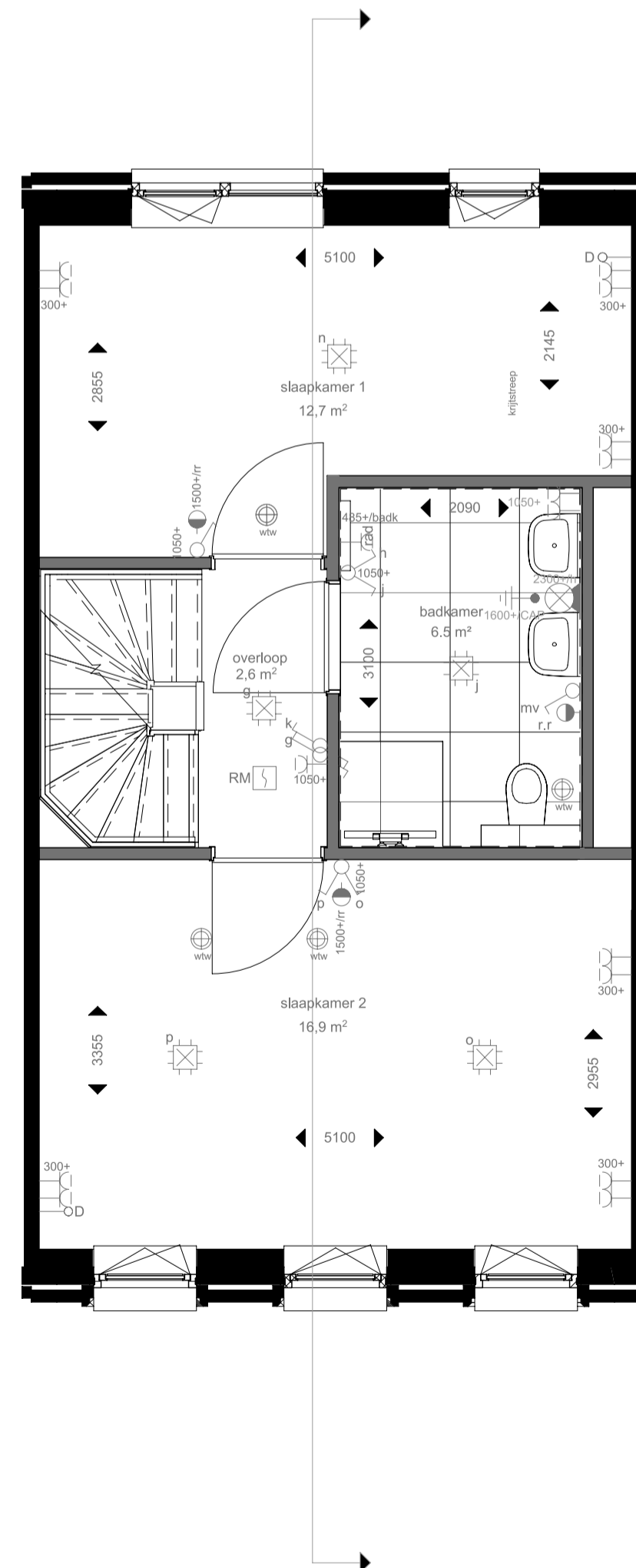
eerste verdieping
