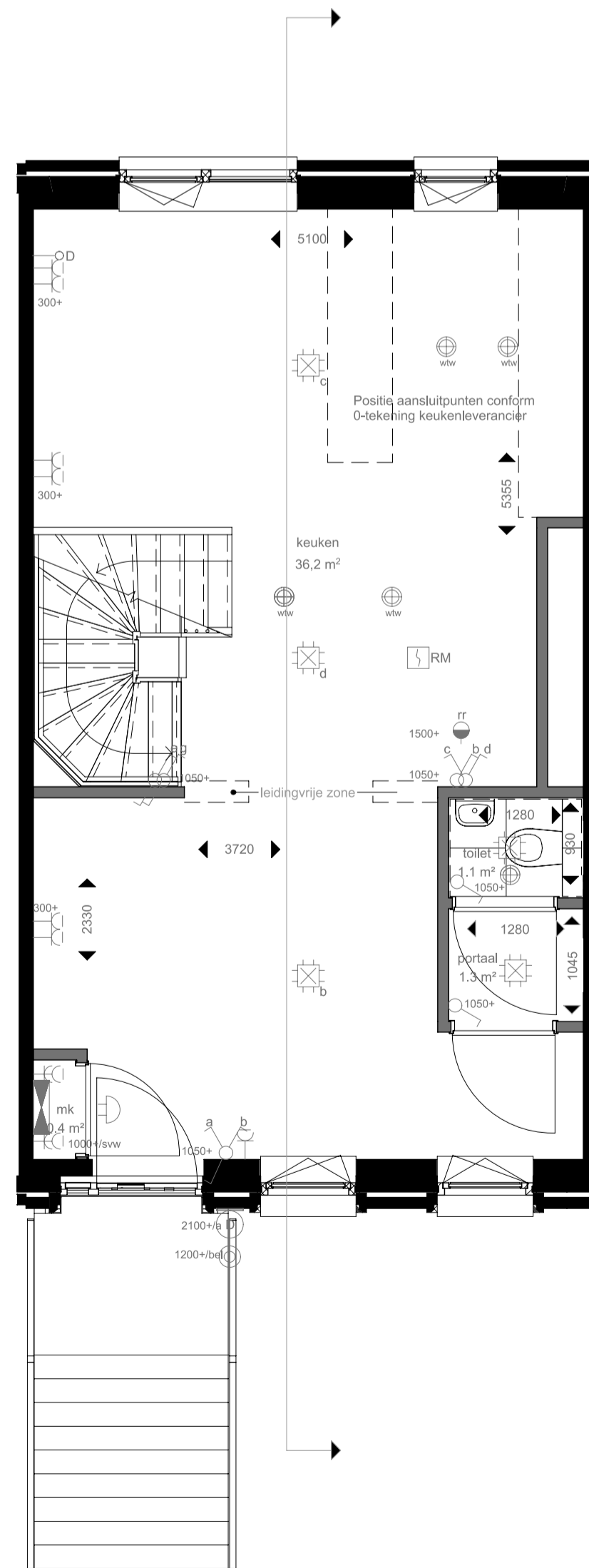
begane grond
