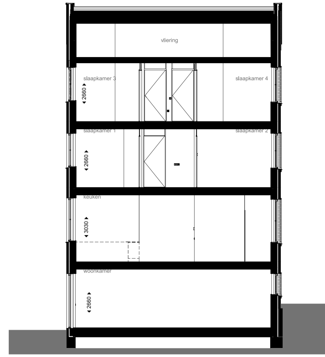
doorsnede
