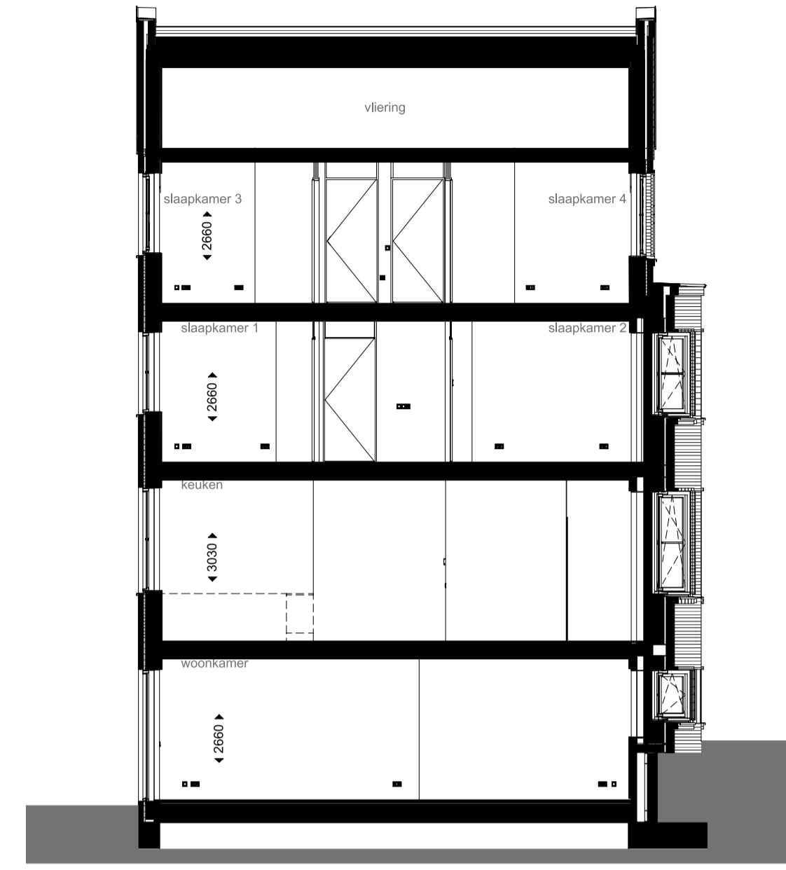
doorsnede
