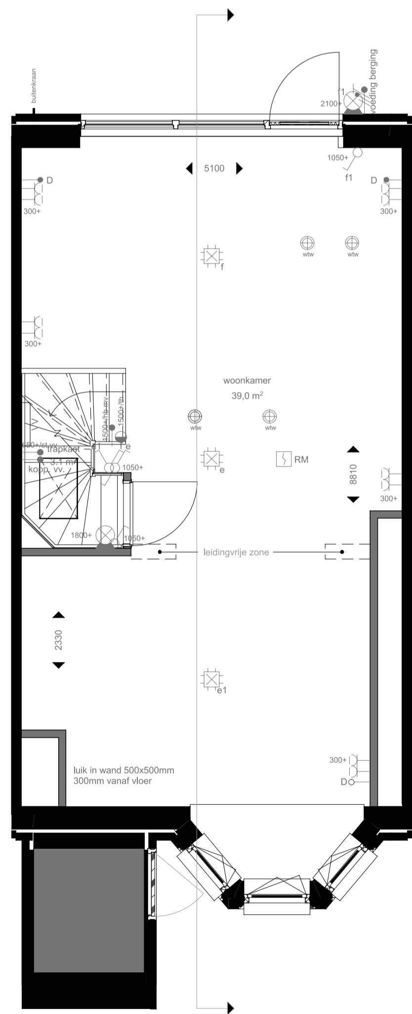
souterrain
