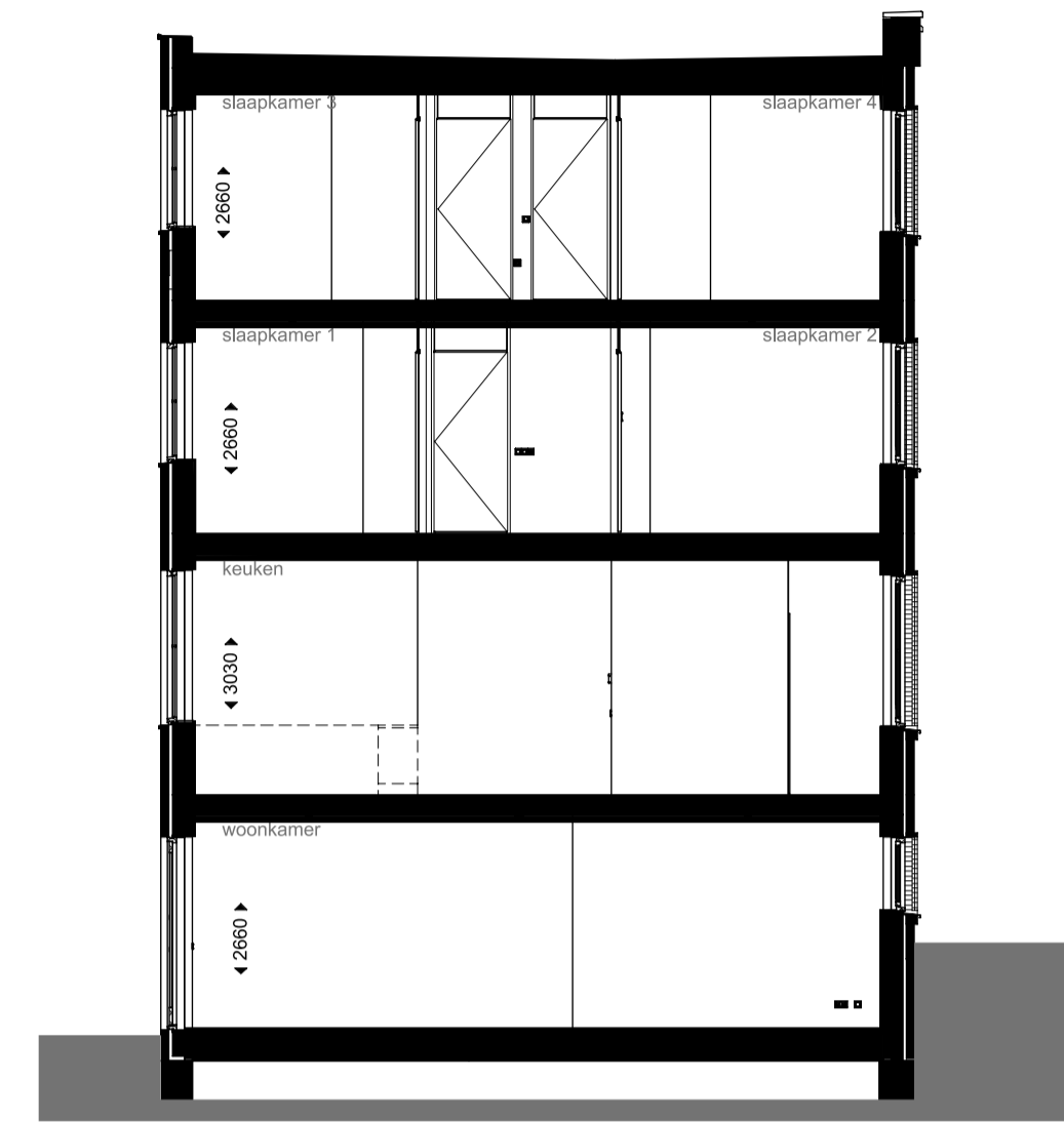
doorsnede
