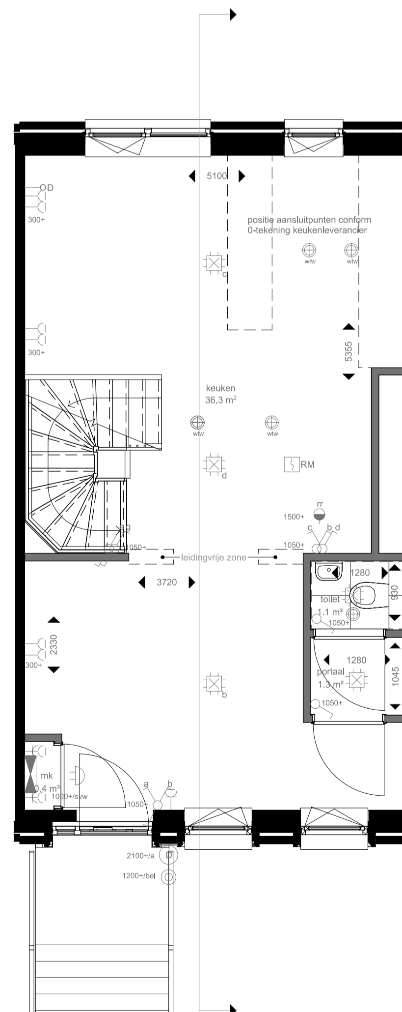
begane grond
