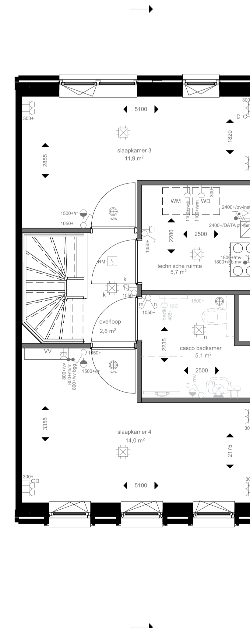
tweede verdieping
