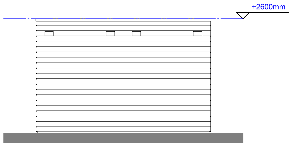
Achteraanzicht 1 : 50
