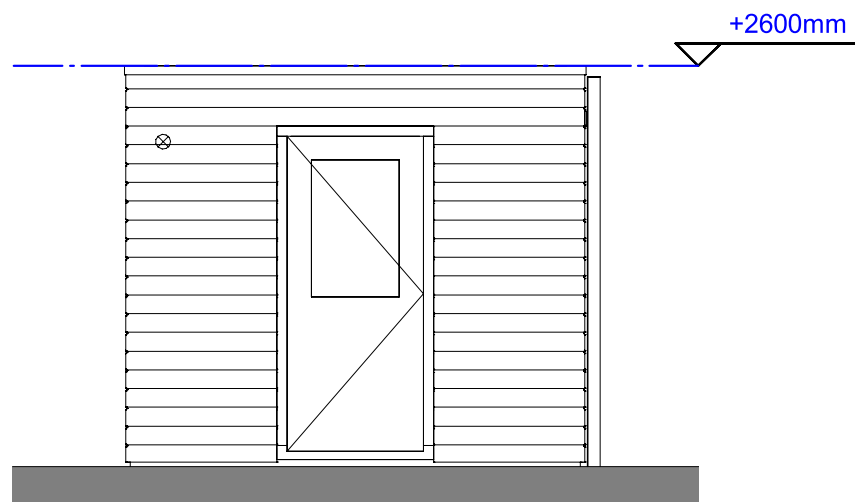
Linker zijaanzicht 1 : 50
