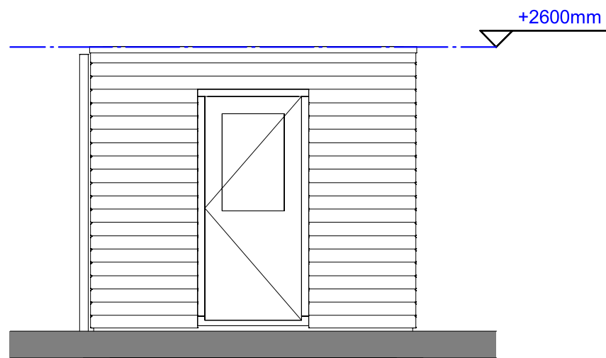
Rechter zijaanzicht 1 : 50
