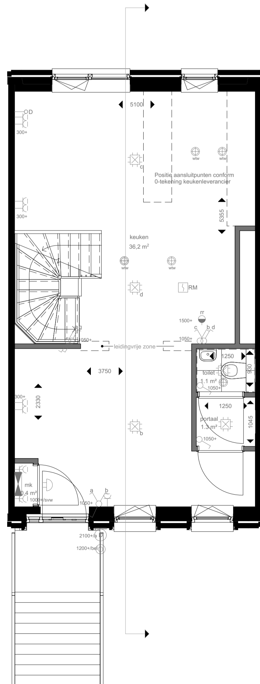
begane grond
