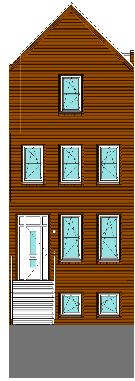
voorgevel
