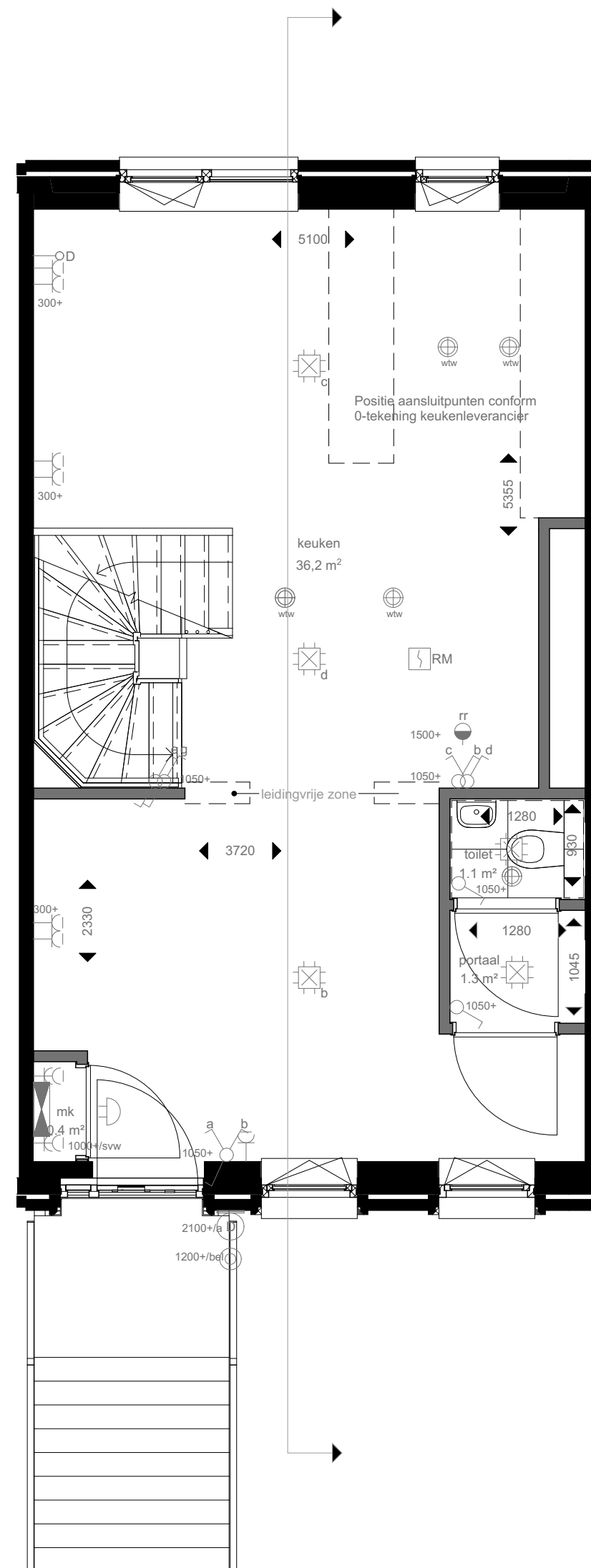
begane grond
