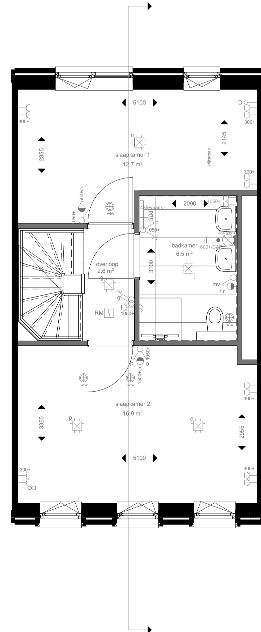
eerste verdieping
