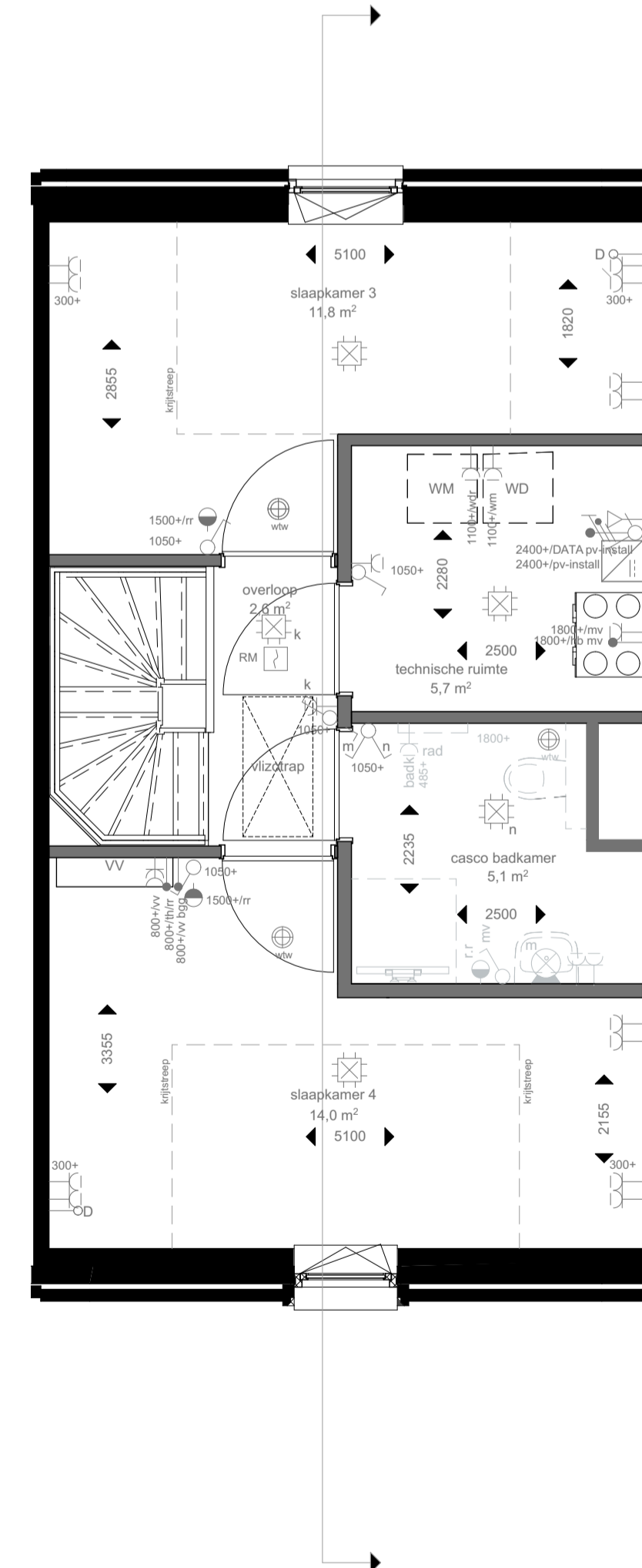
tweede verdieping
