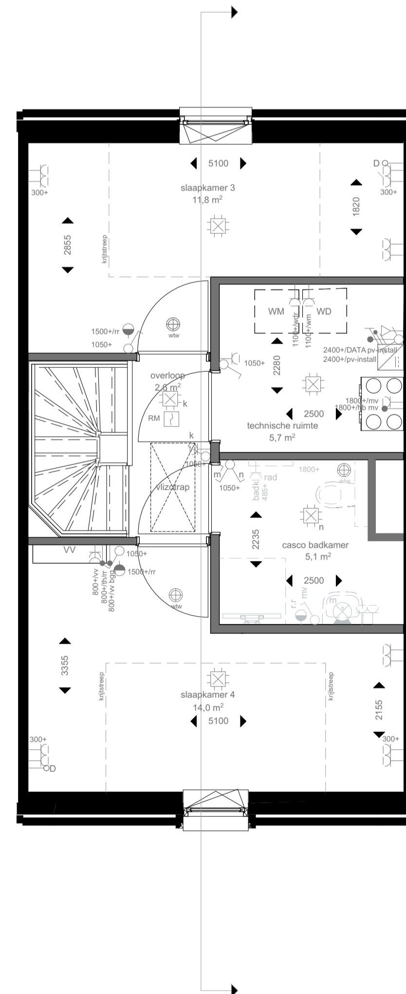
tweede verdieping
