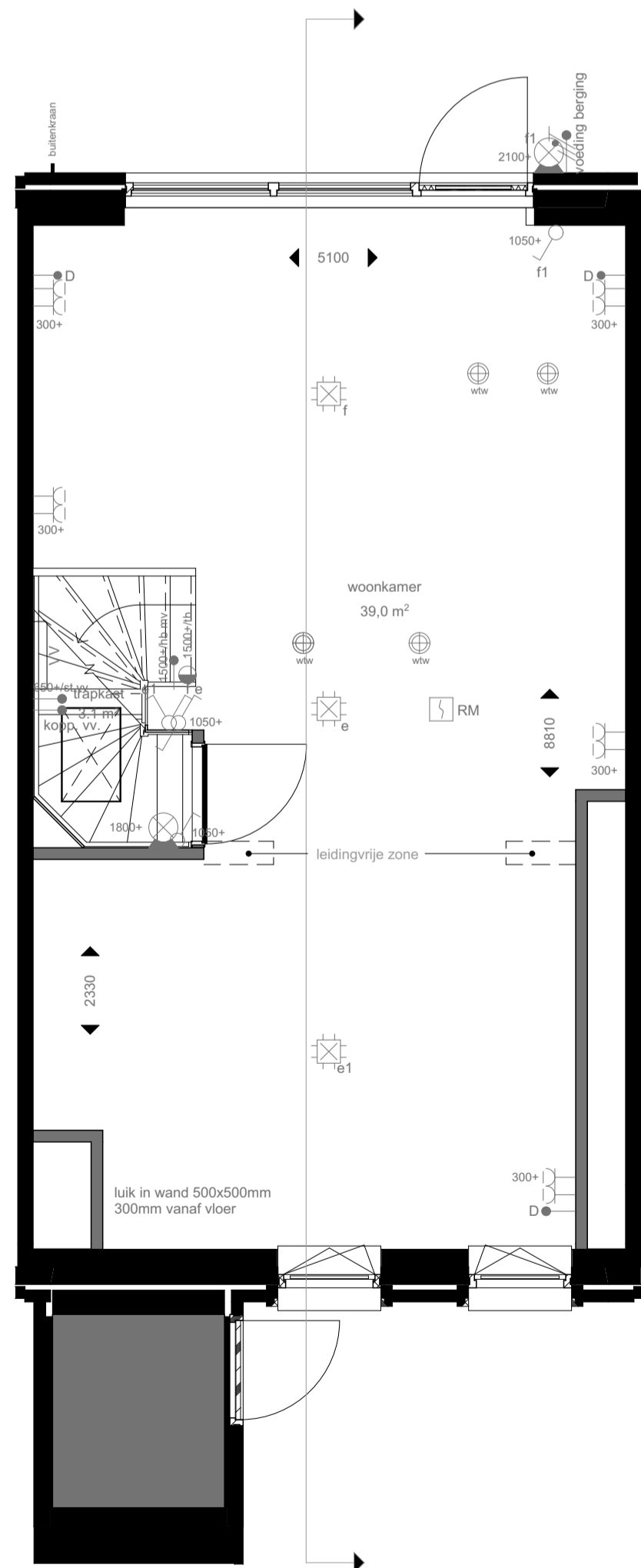
souterrain
