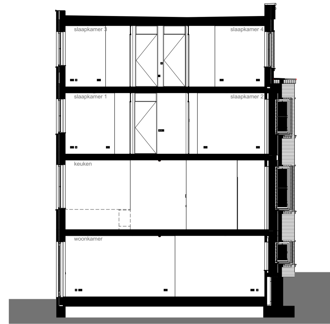
doorsnede
