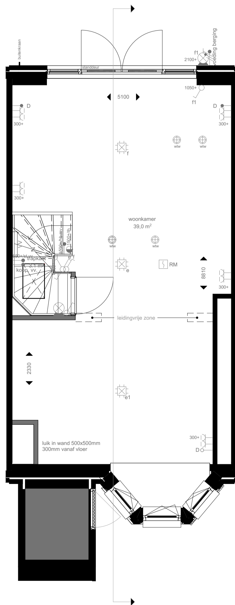
souterrain
