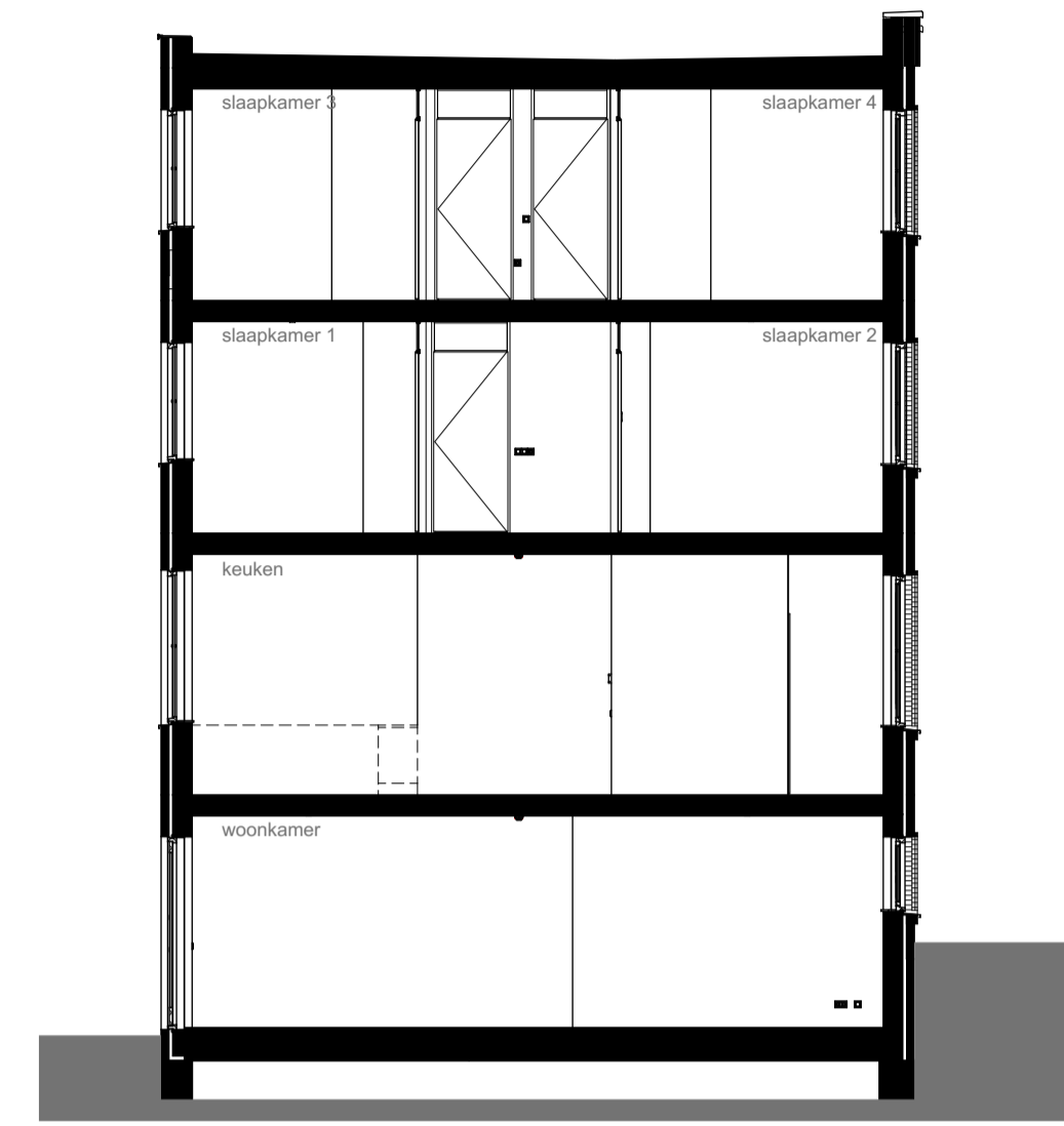
doorsnede
