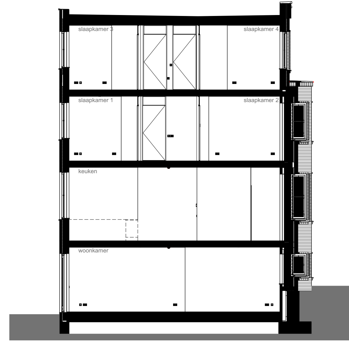
doorsnede
