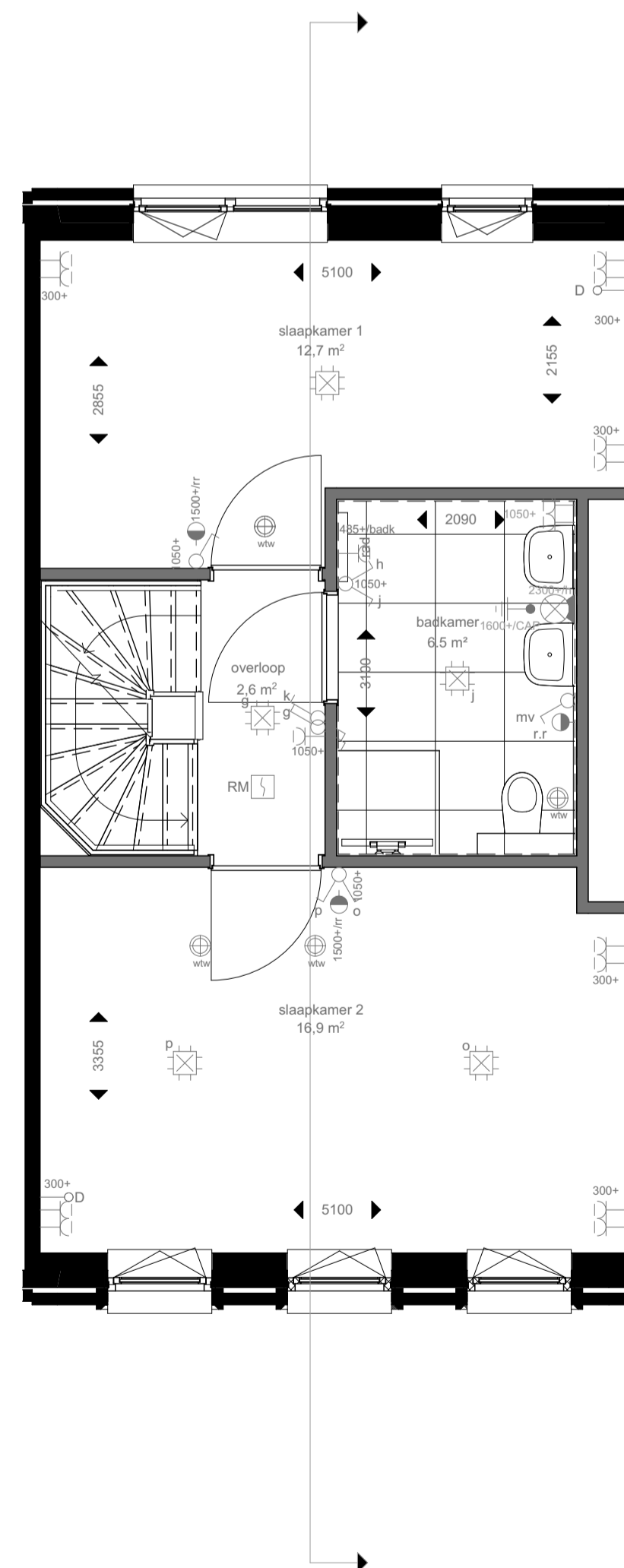
eerste verdieping
