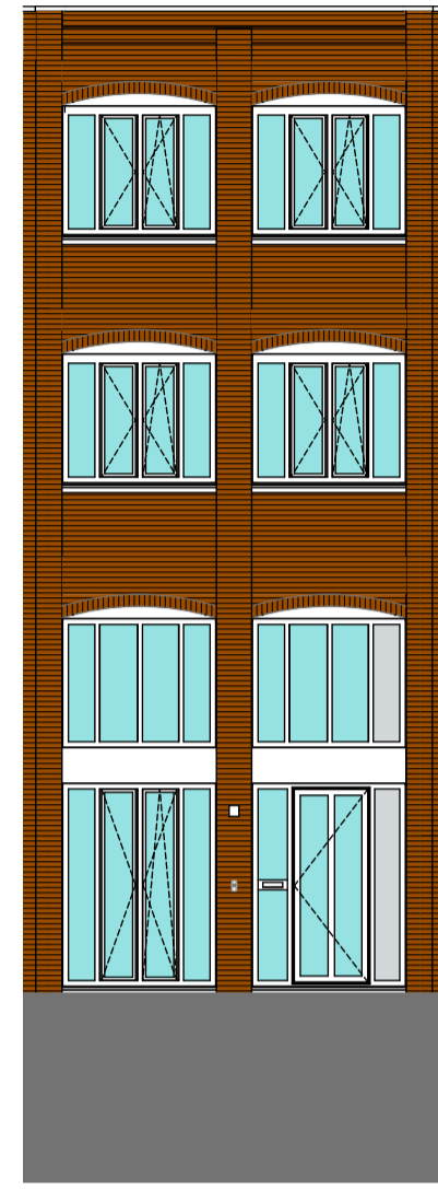
voorgevel
