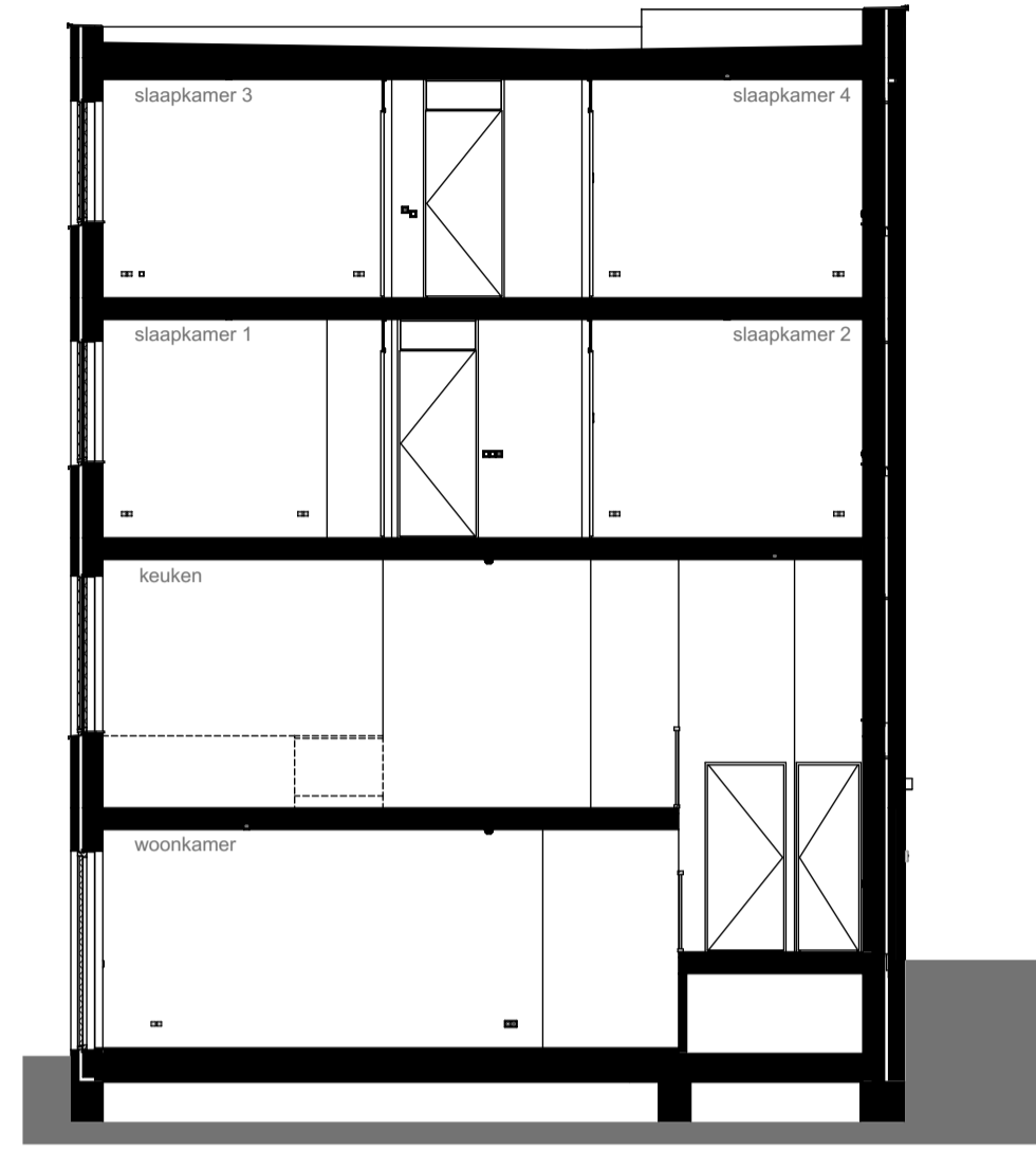
doorsnede
