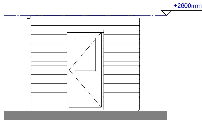
Rechter zijaanzicht
