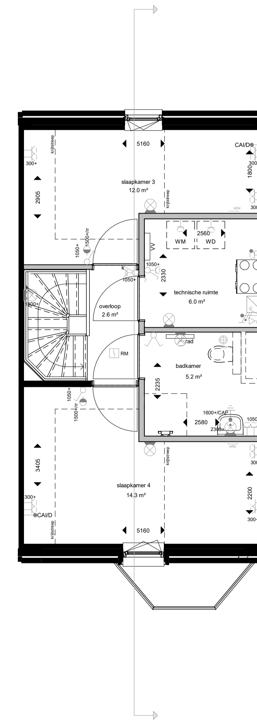
tweede verdieping
