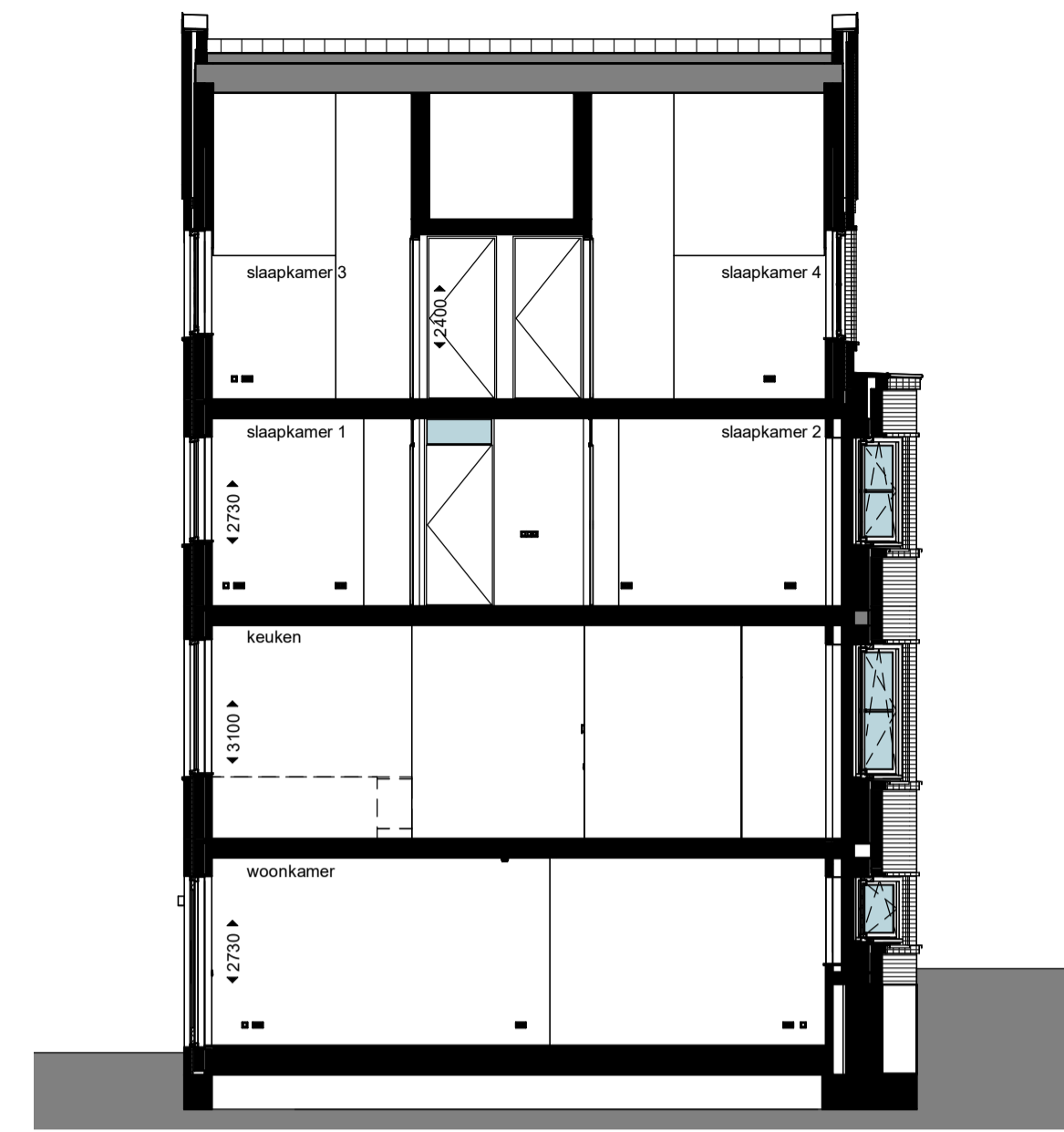
doorsnede
