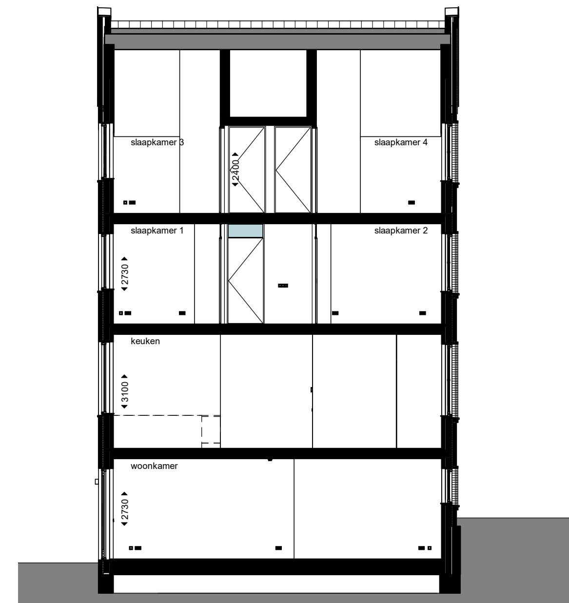
doorsnede
