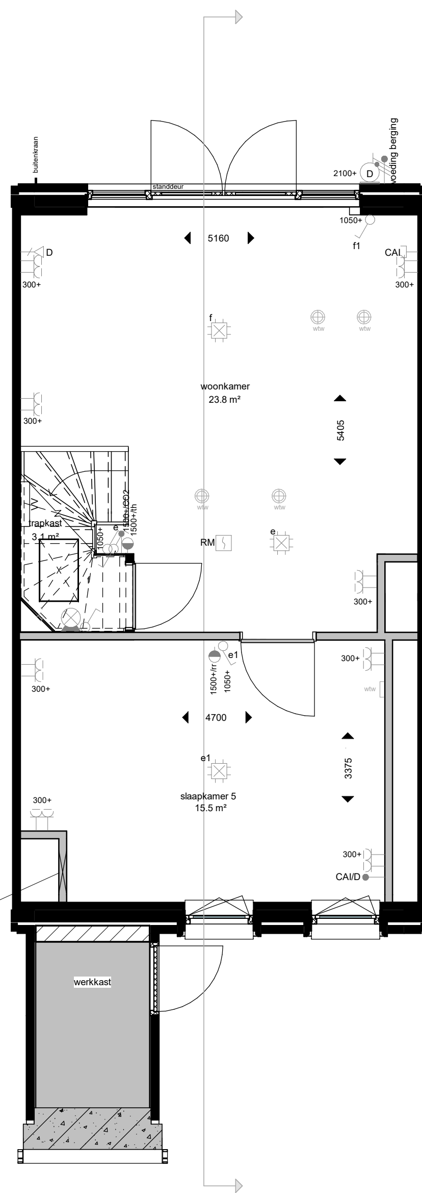
souterrain
