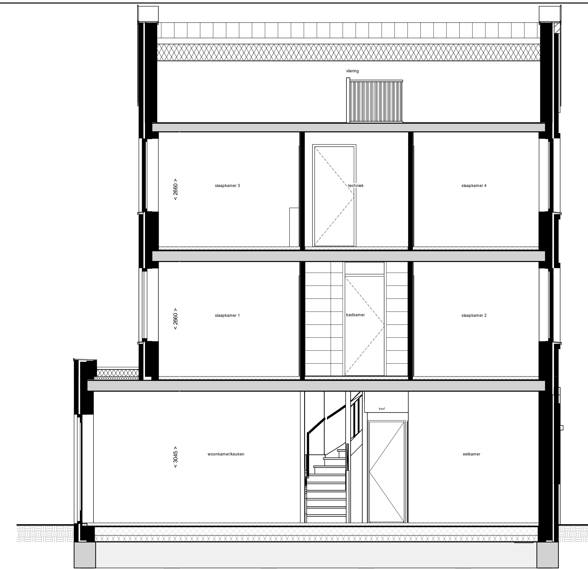
Doorsnede C09
