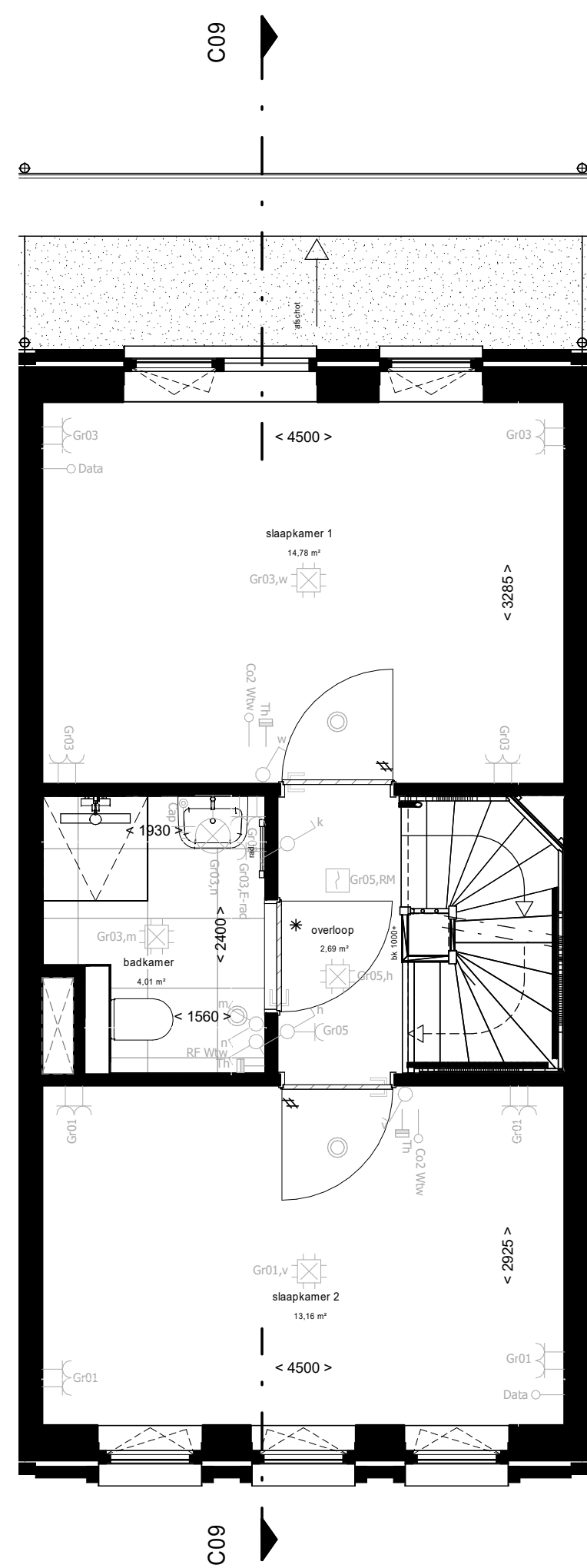
1e verdieping
