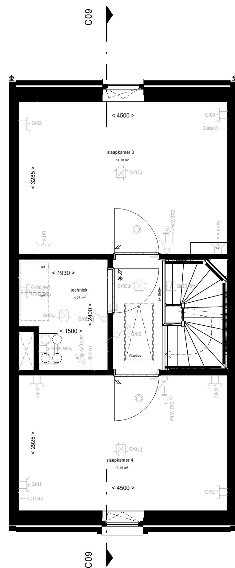
2e verdieping
