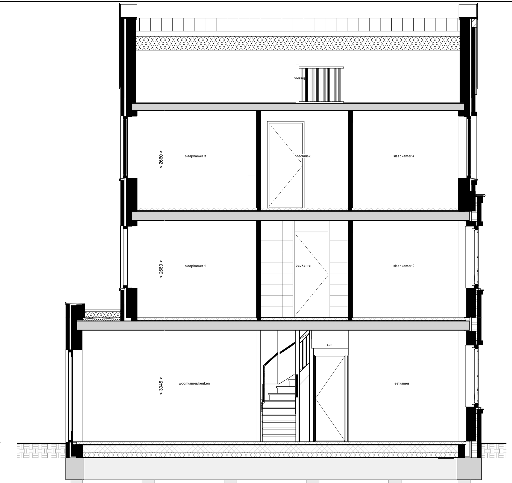
Doorsnede C08
