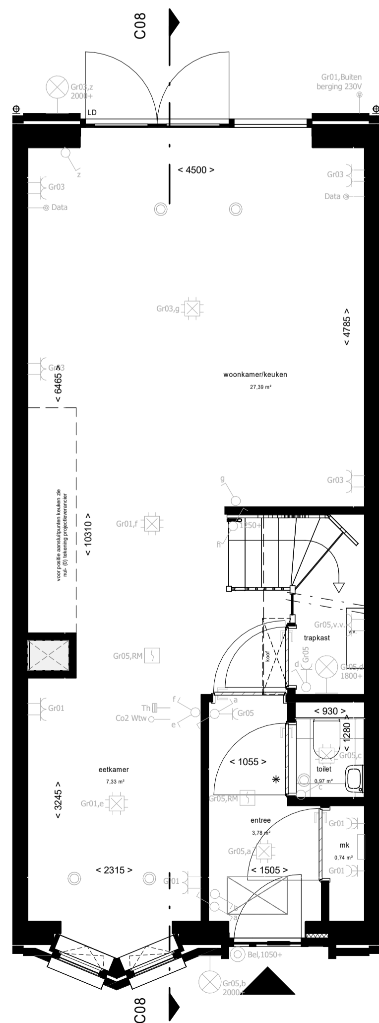
Begane grond
