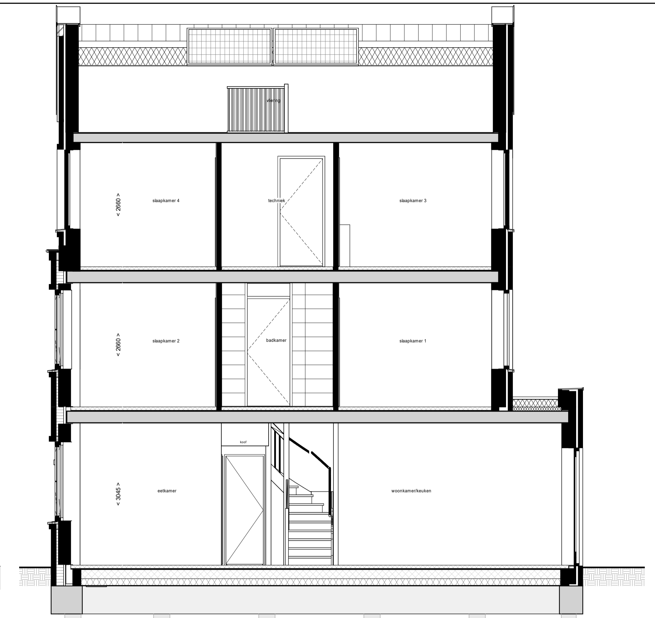
Doorsnede V07
