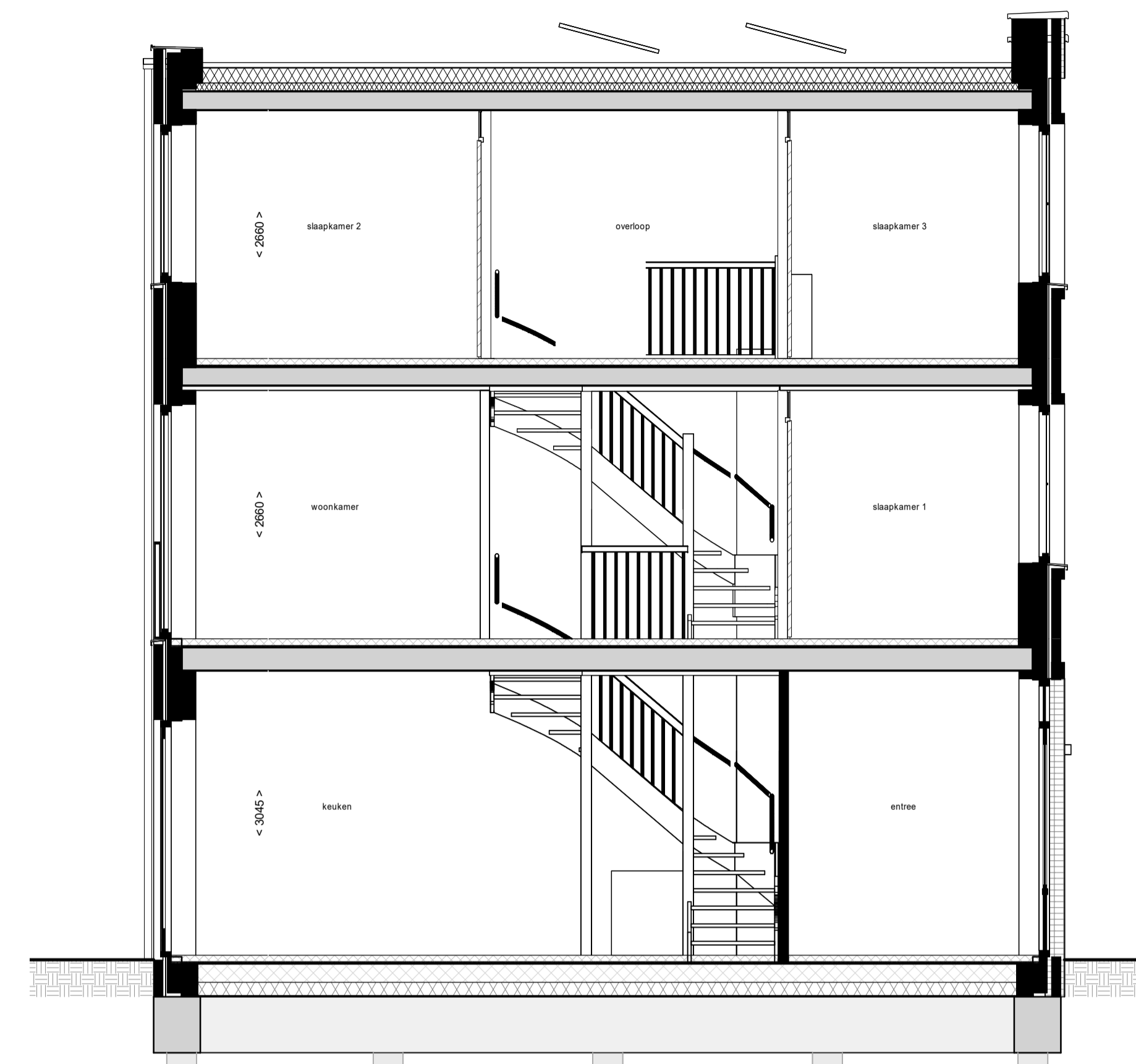
Doorsnede C06
