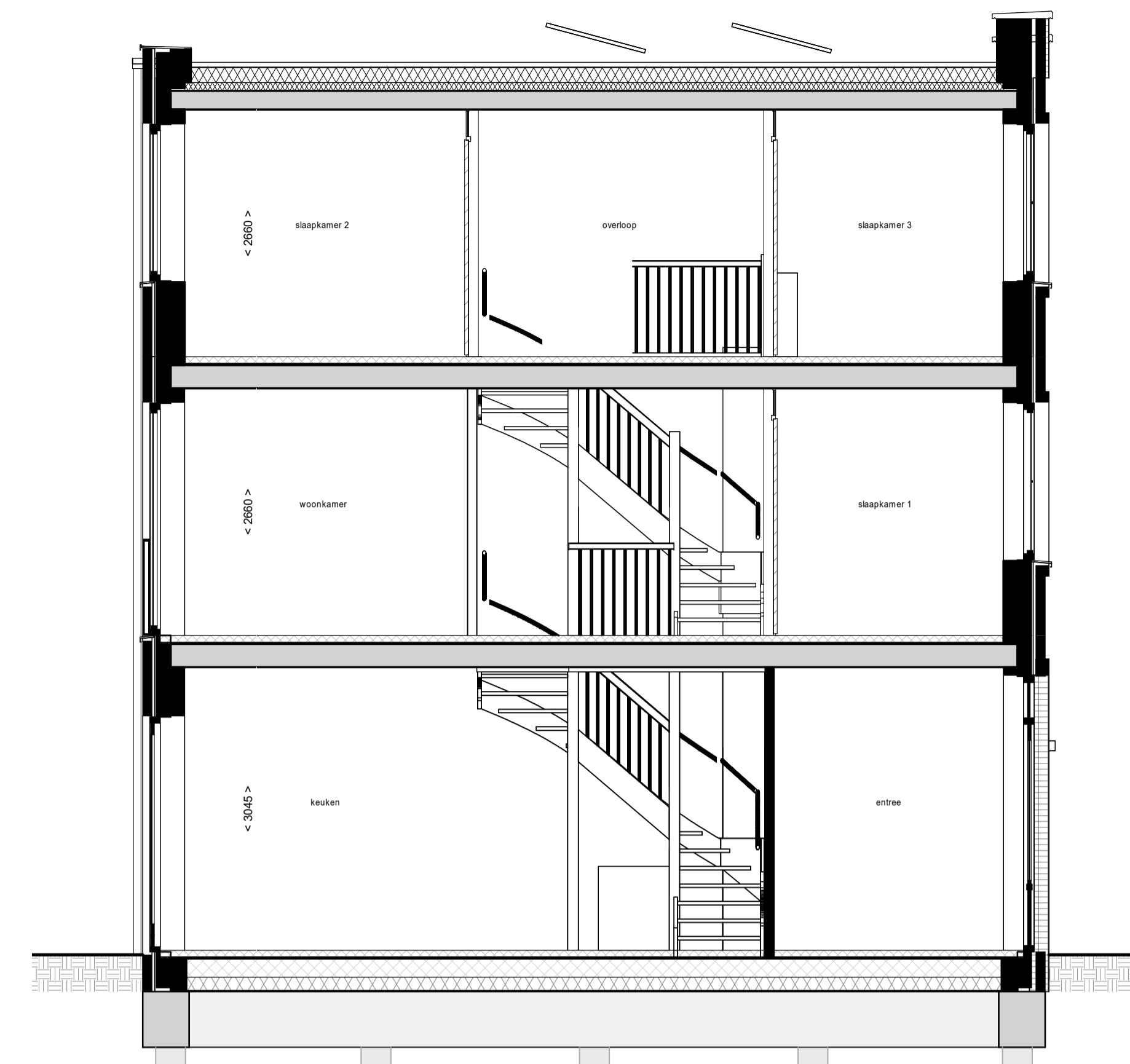
Doorsnede C05
