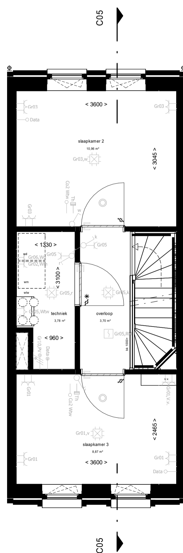
2e verdieping
