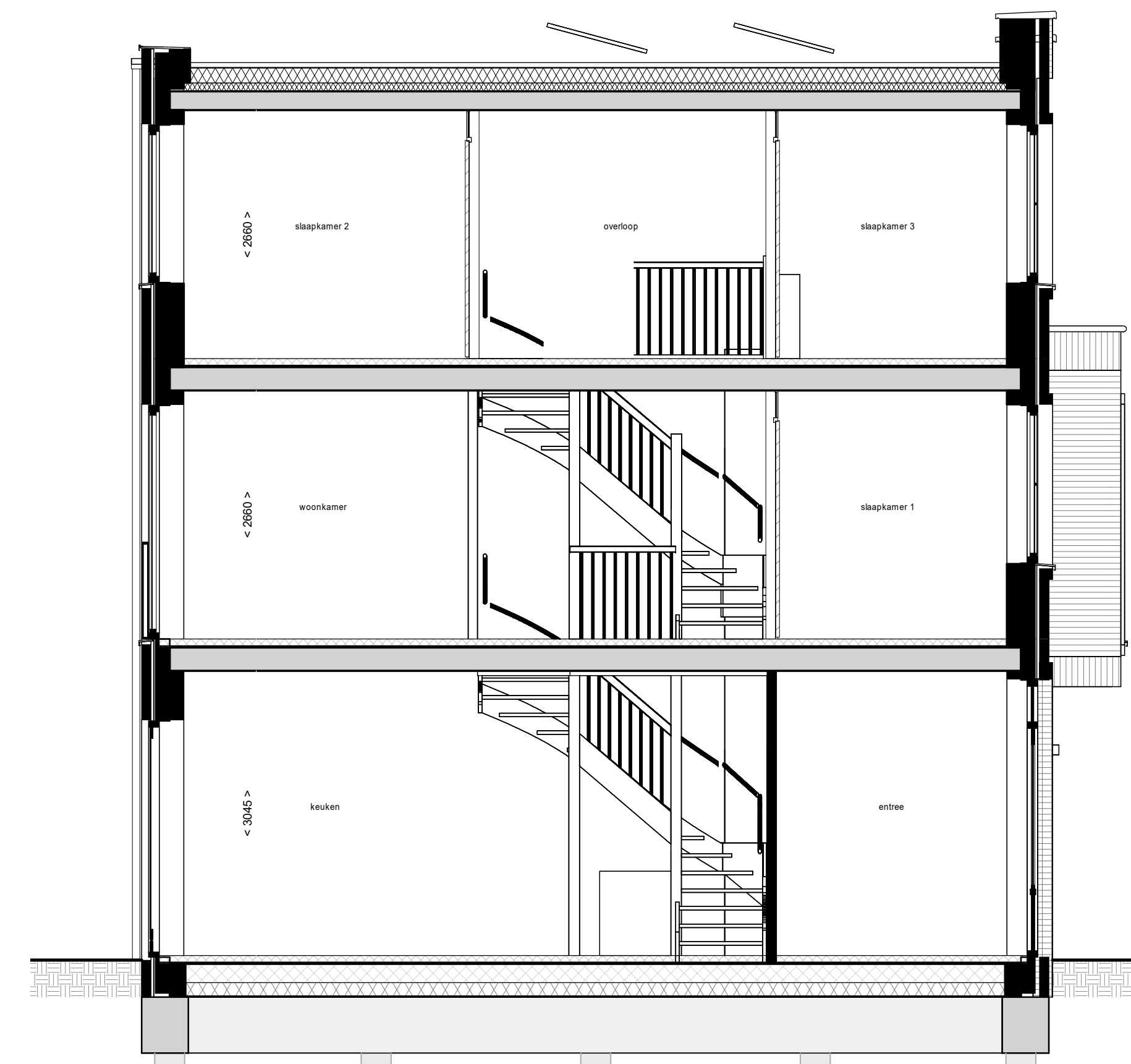
Doorsnede C04
