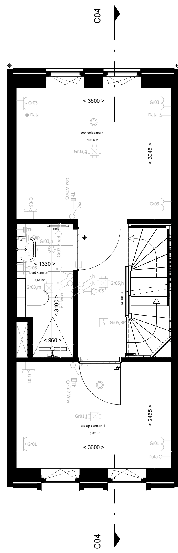
1e verdieping
