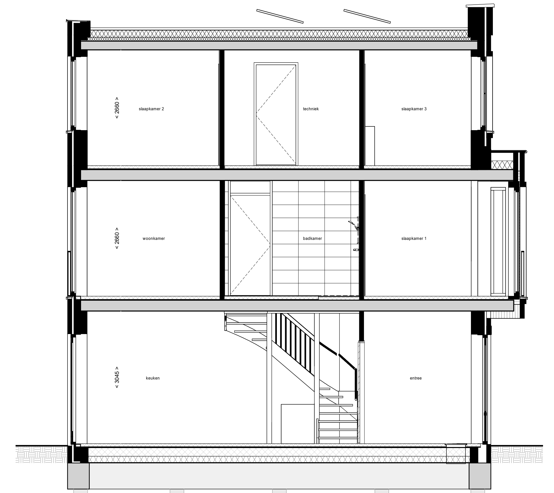
Doorsnede C03
