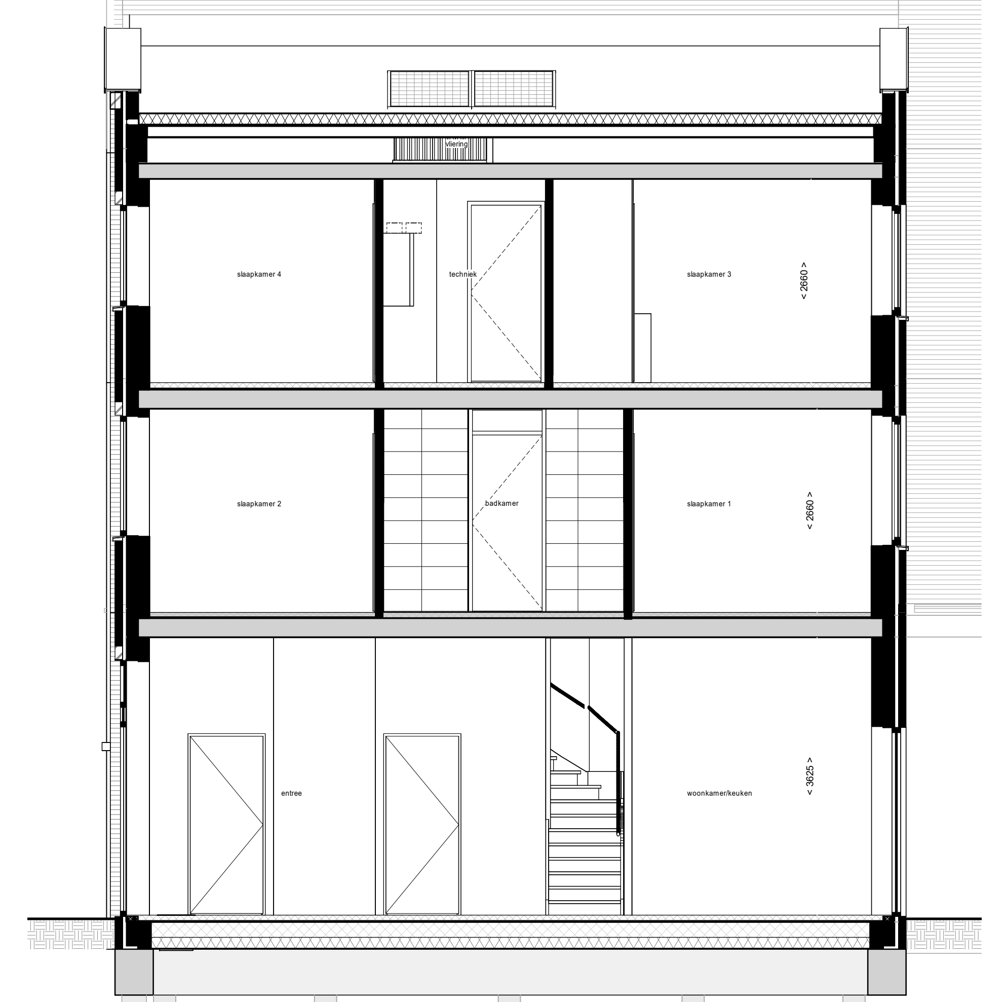
Doorsnede B22
