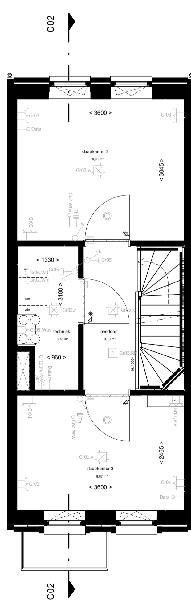
2e verdieping
