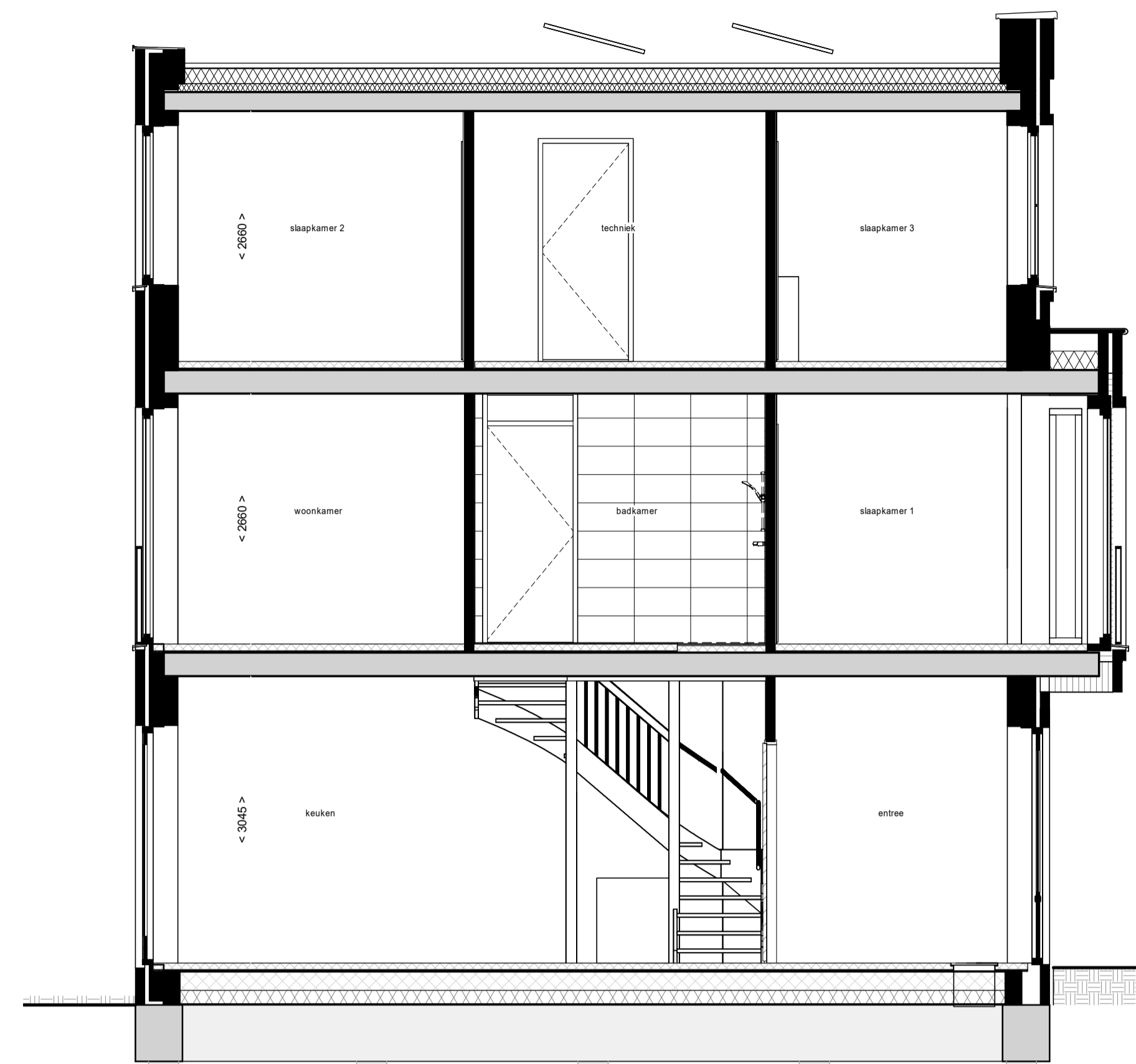
Doorsnede C02
