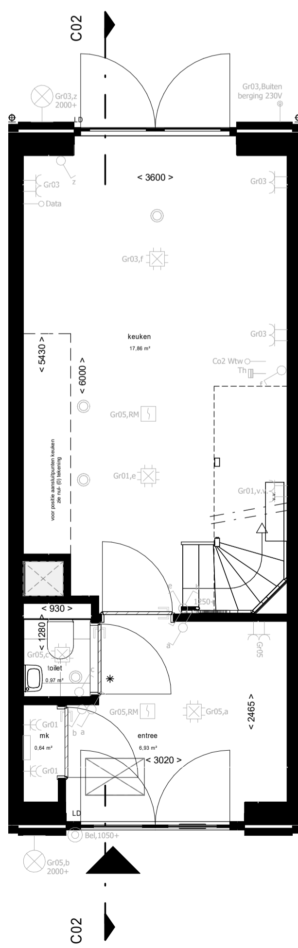
Begane grond
