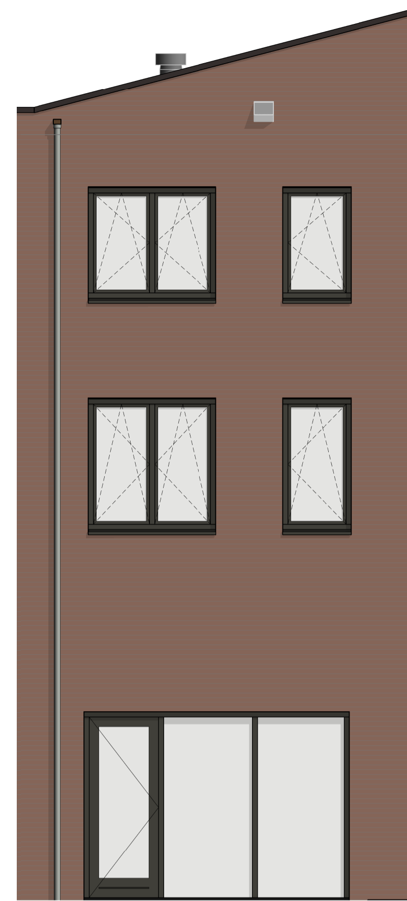
Achtergevel
