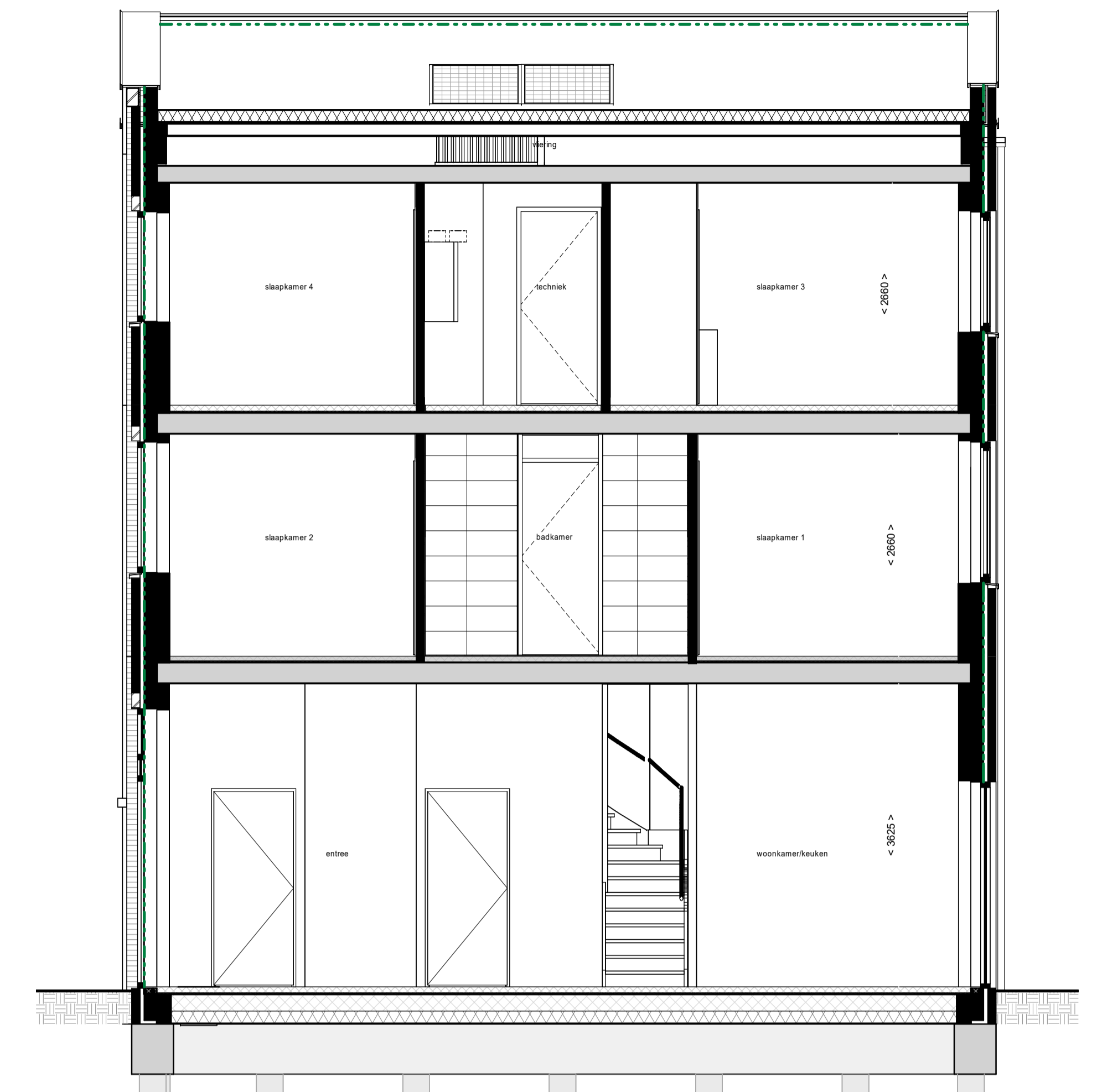
Doorsnede B19
