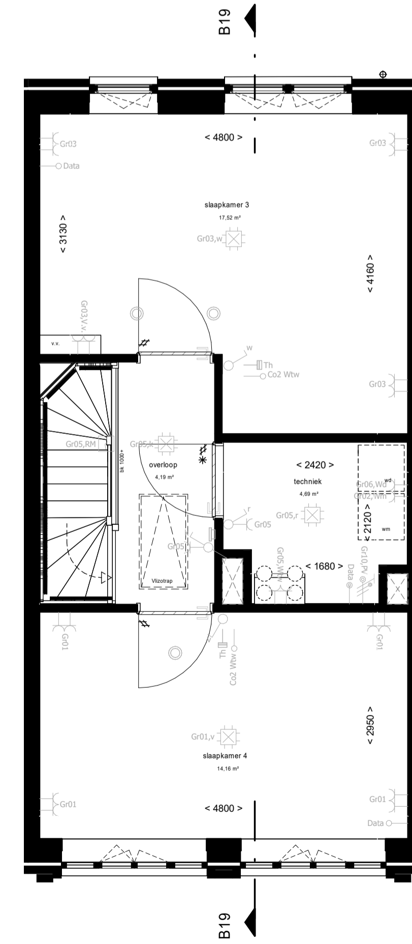
2e verdieping
