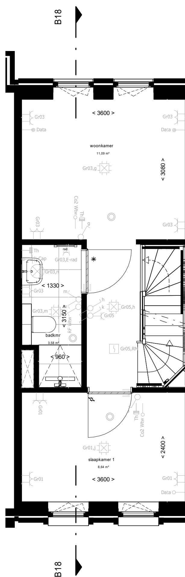
1e verdieping
