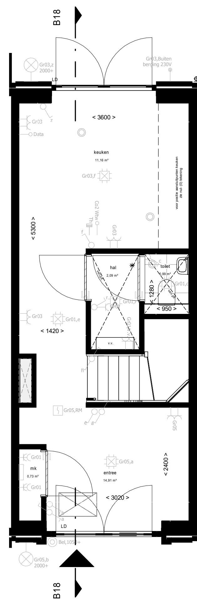
Begane grond
