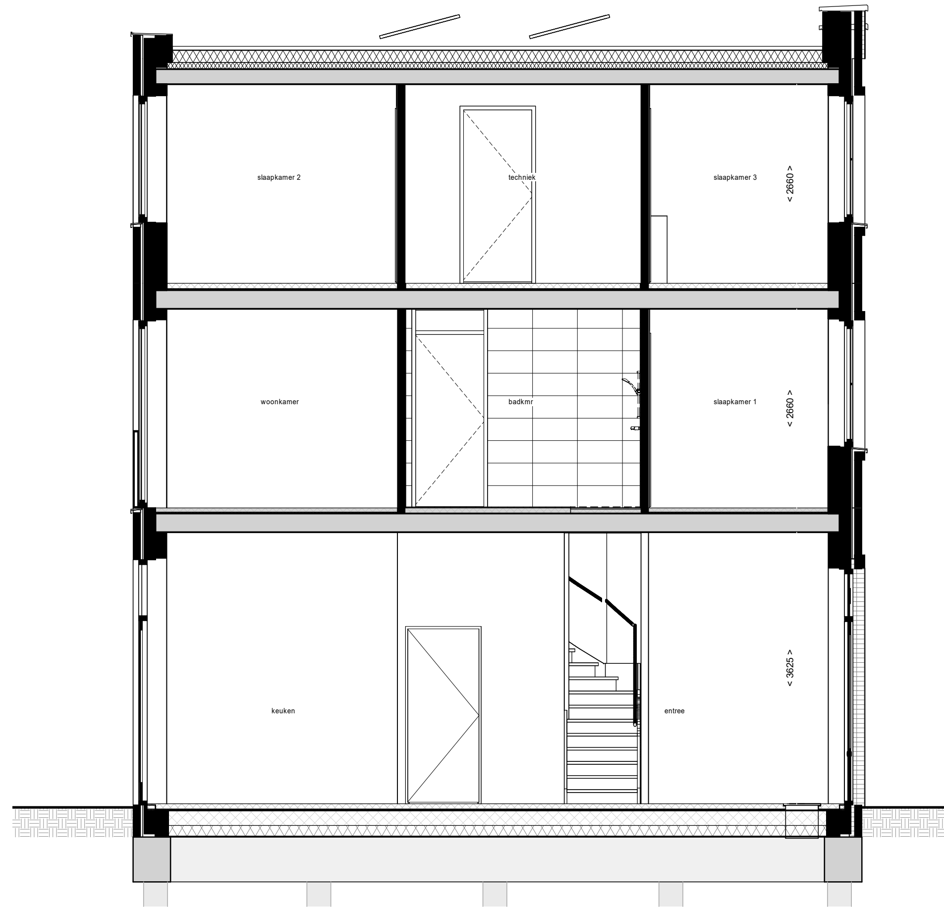
Doorsnede B18
