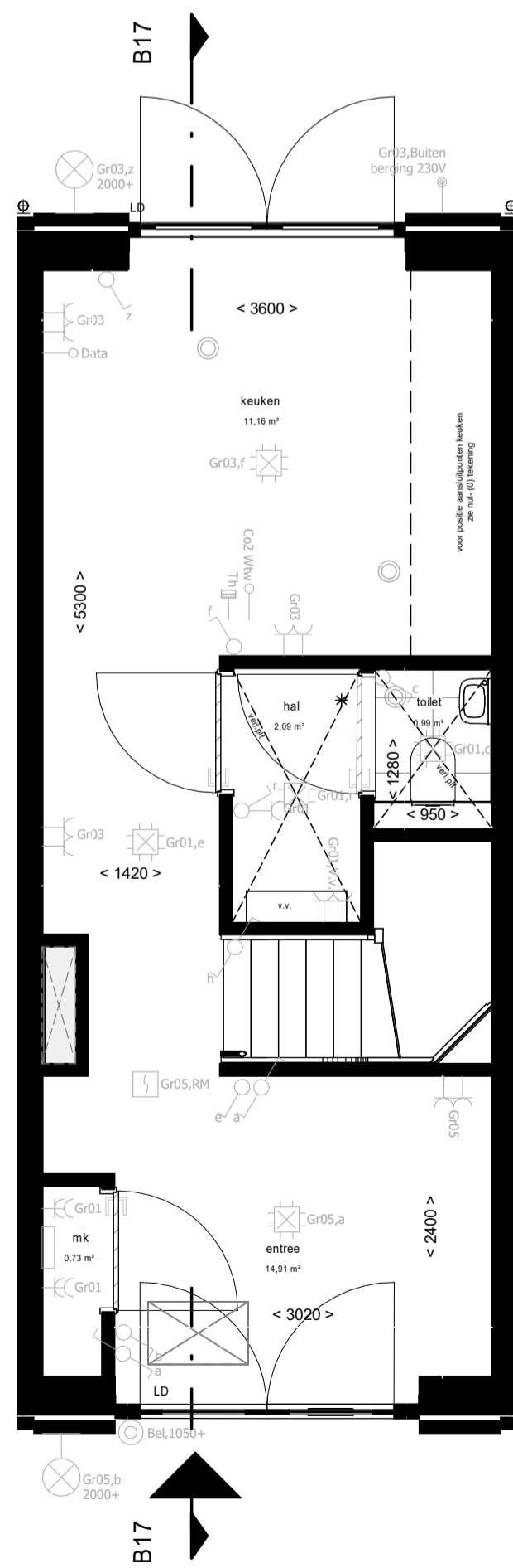
Begane grond
