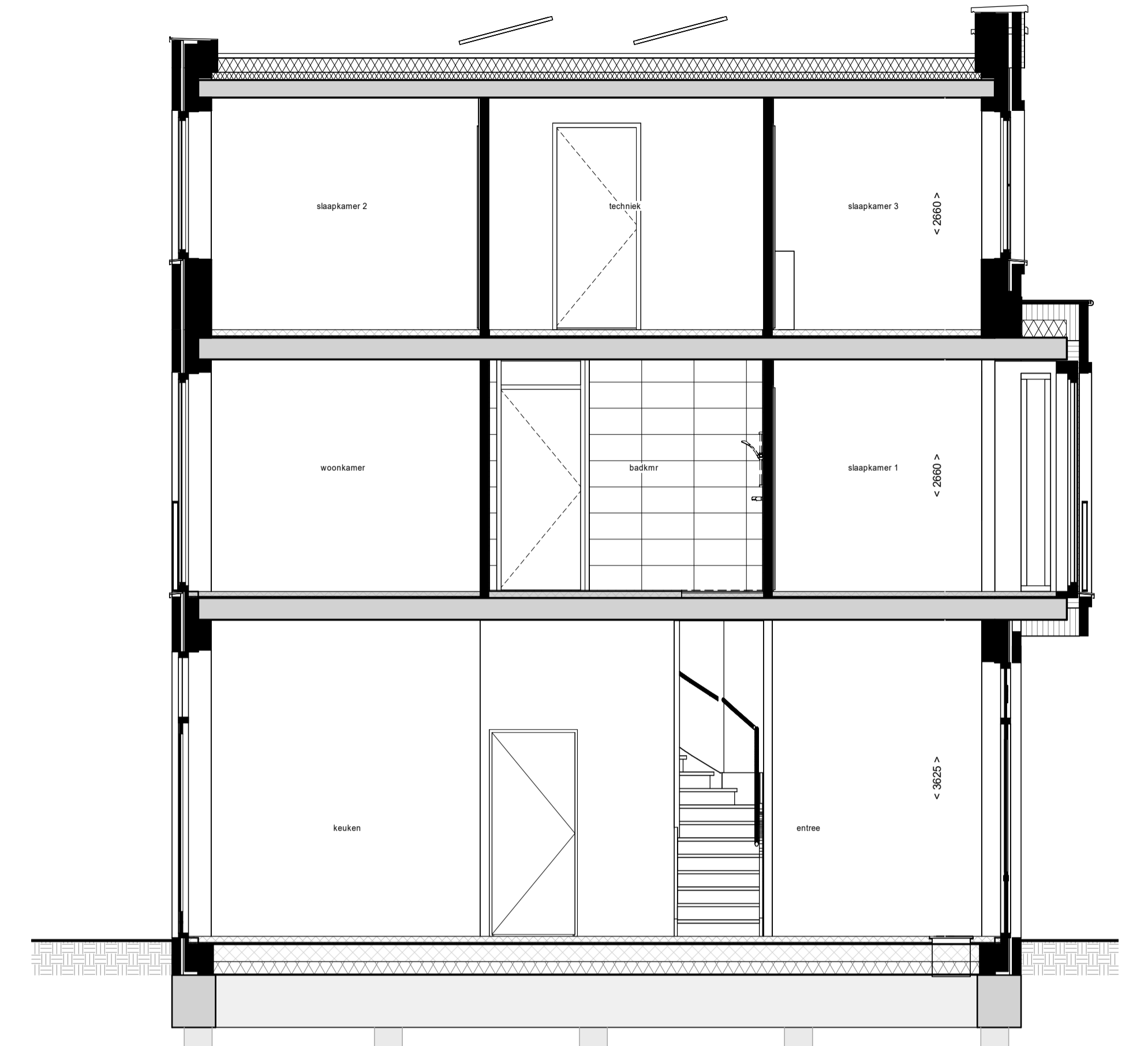
Doorsnede B17
