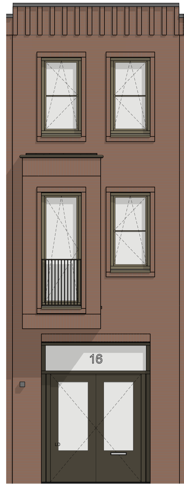
Voorgevel
