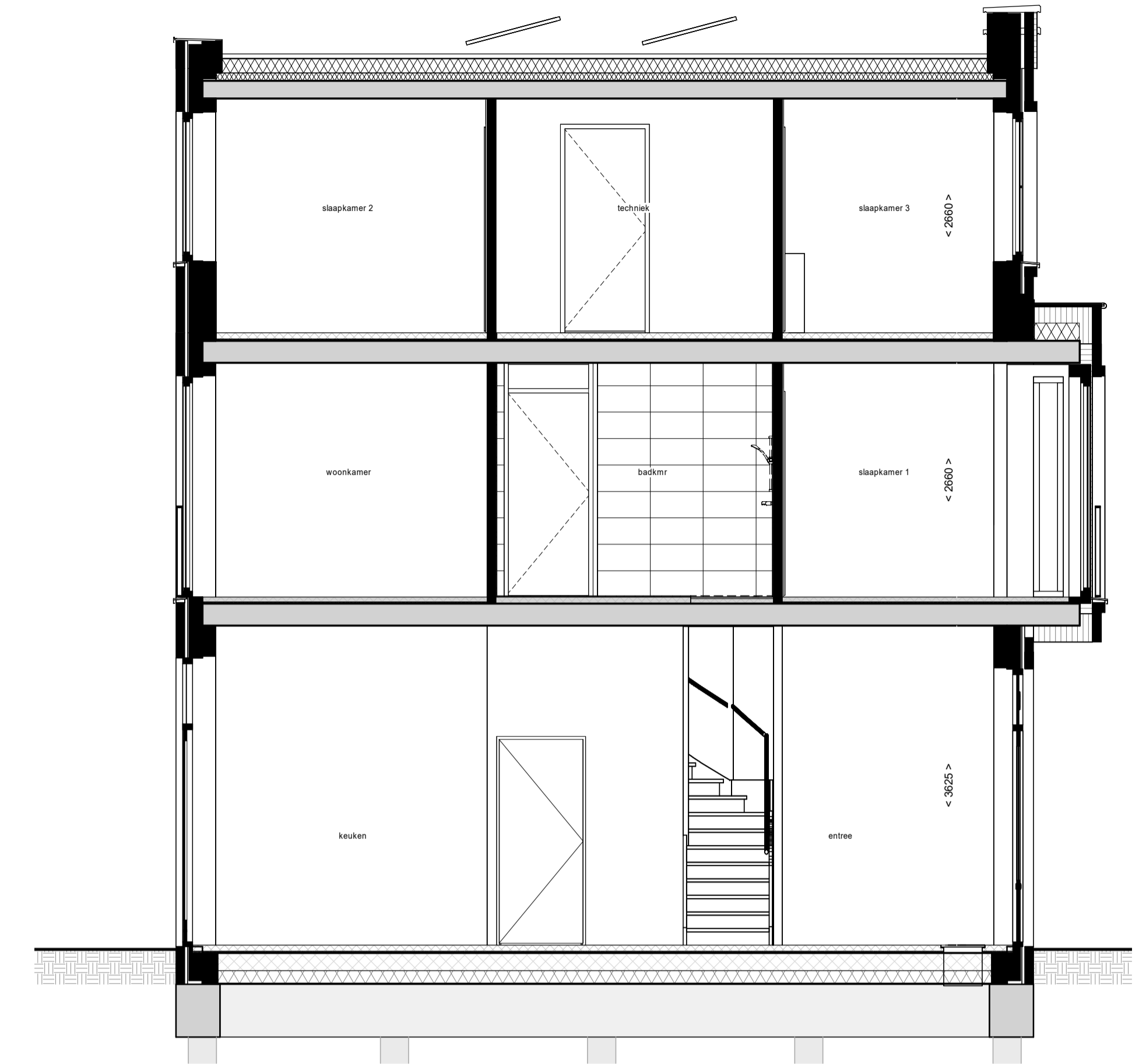
Doorsnede B16
