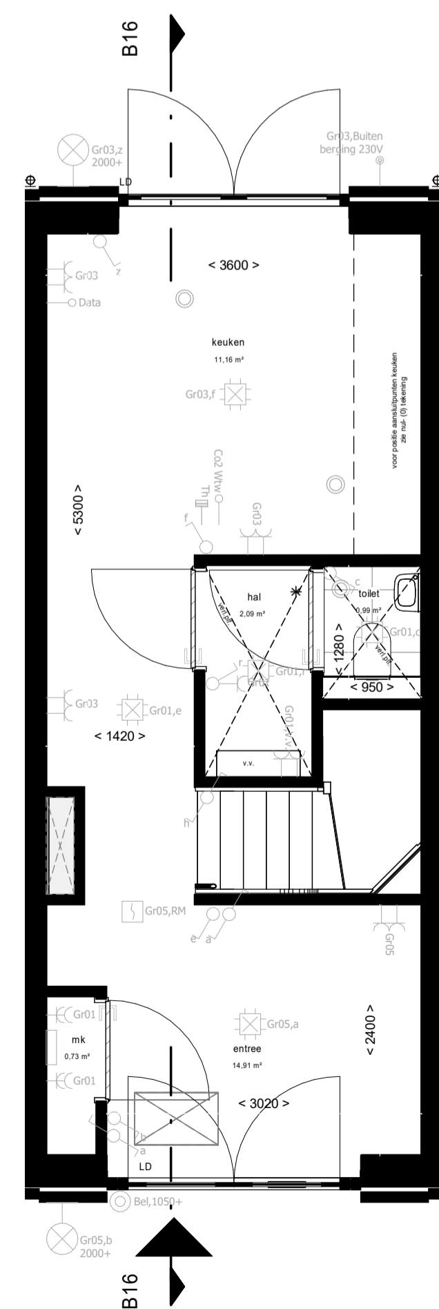
Begane grond
