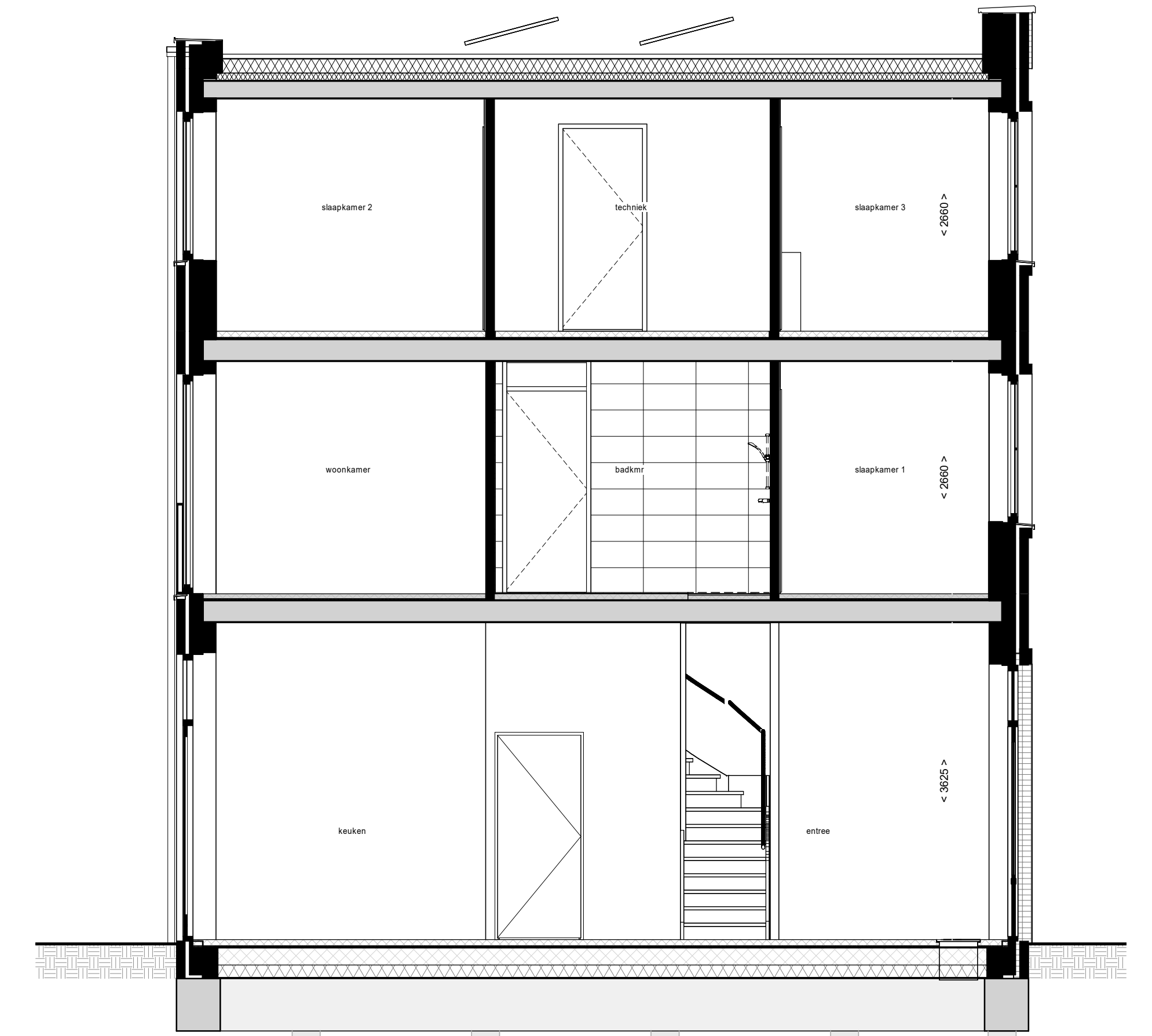
Doorsnede B15
