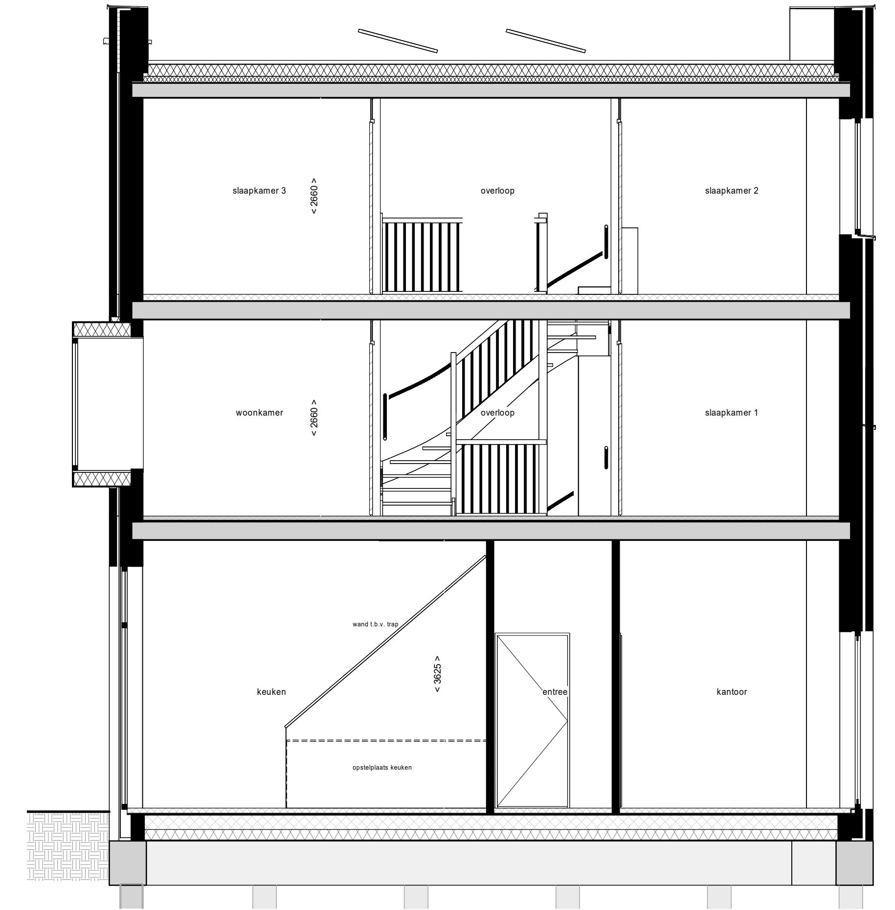
Doorsnede B14
