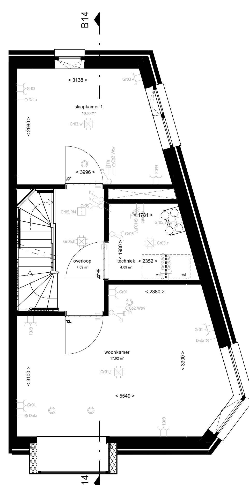
1e verdieping
