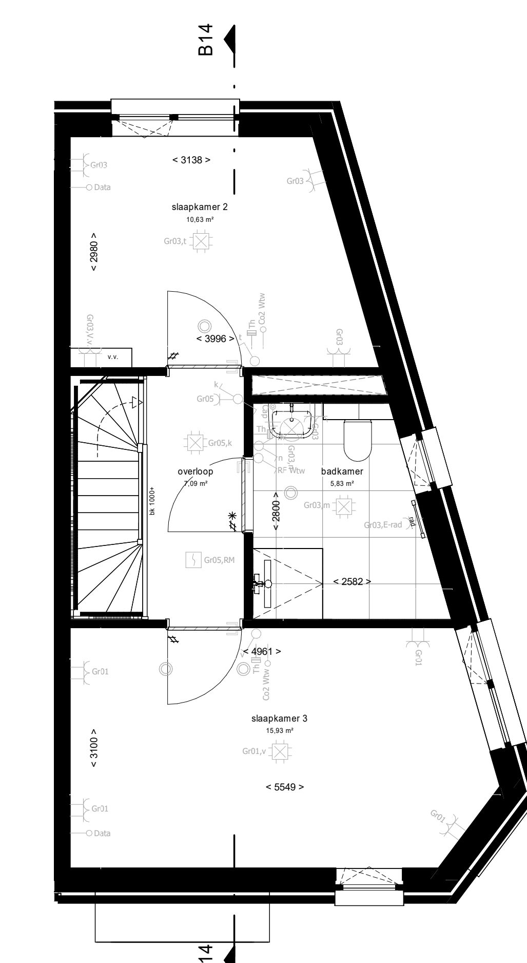
2e verdieping
