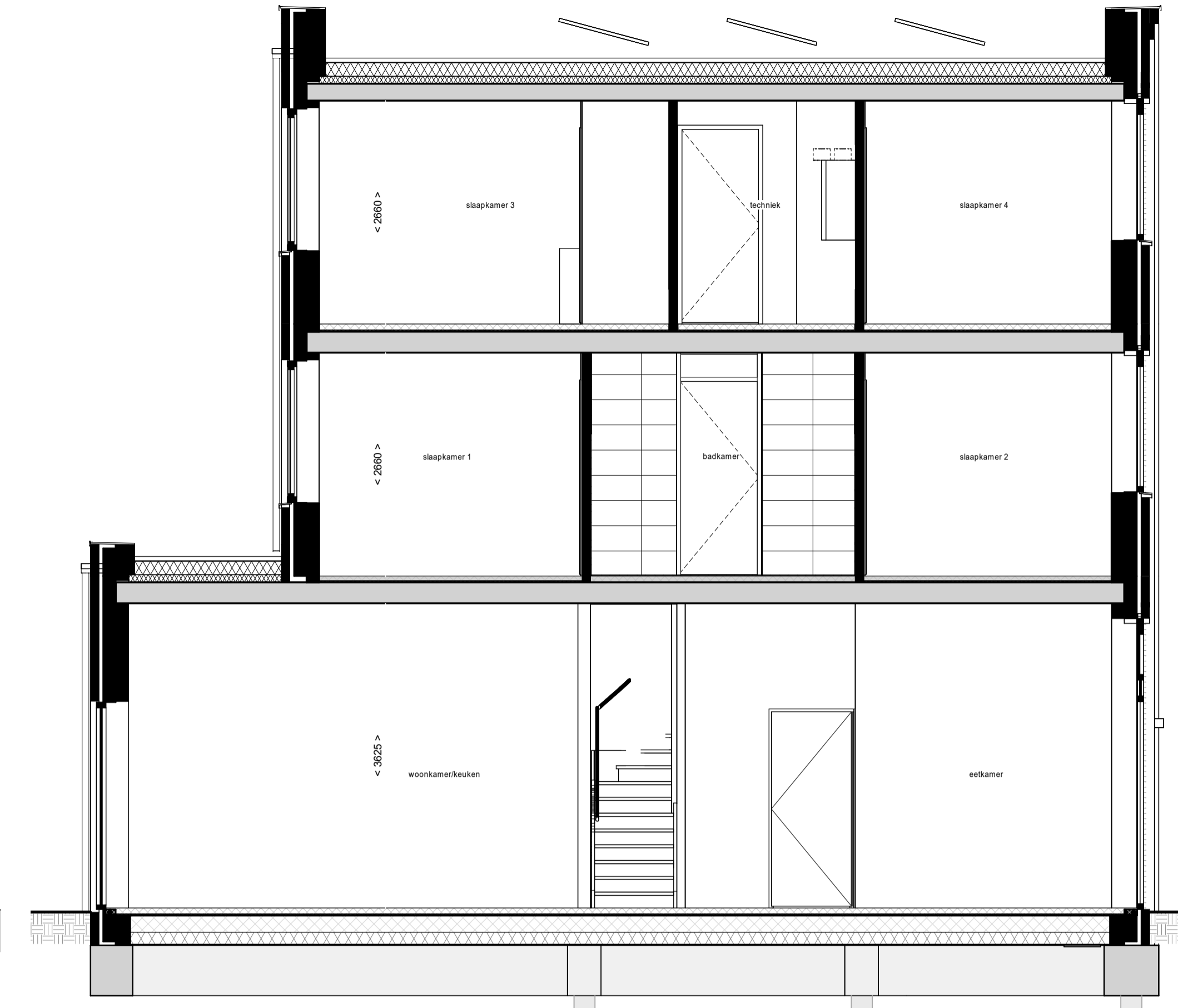
Doorsnede C13
