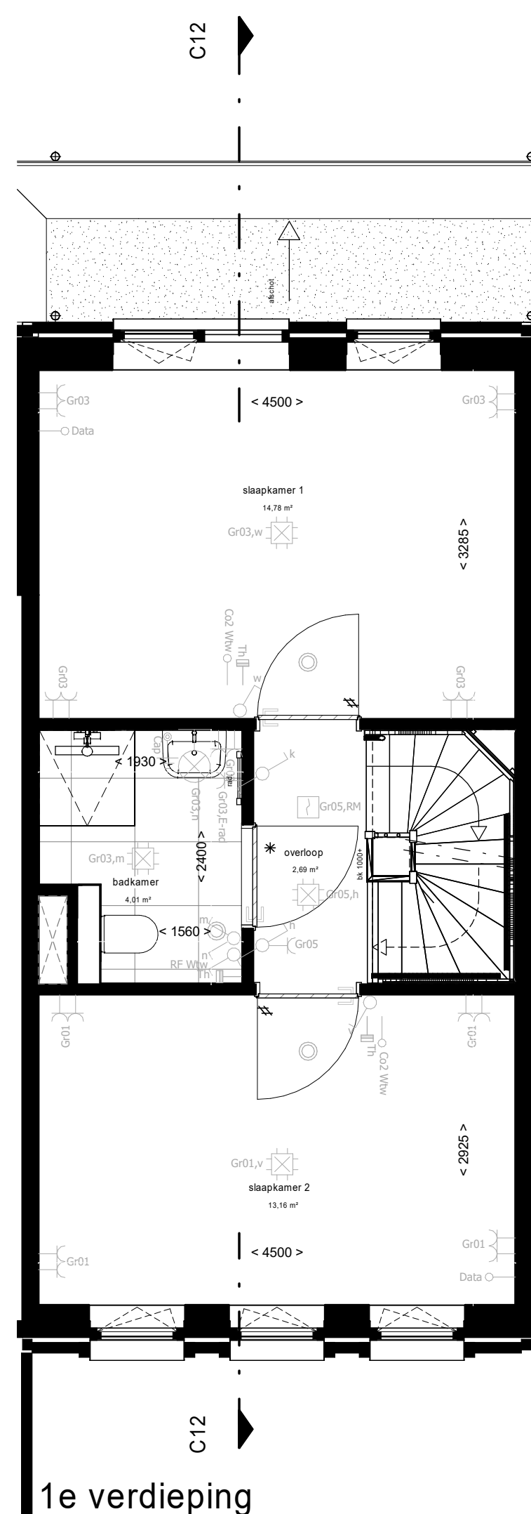
1e verdieping
