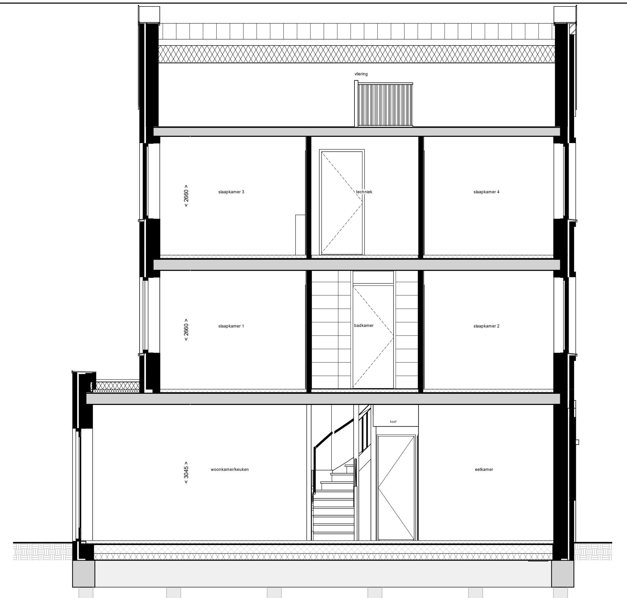
Doorsnede C12
