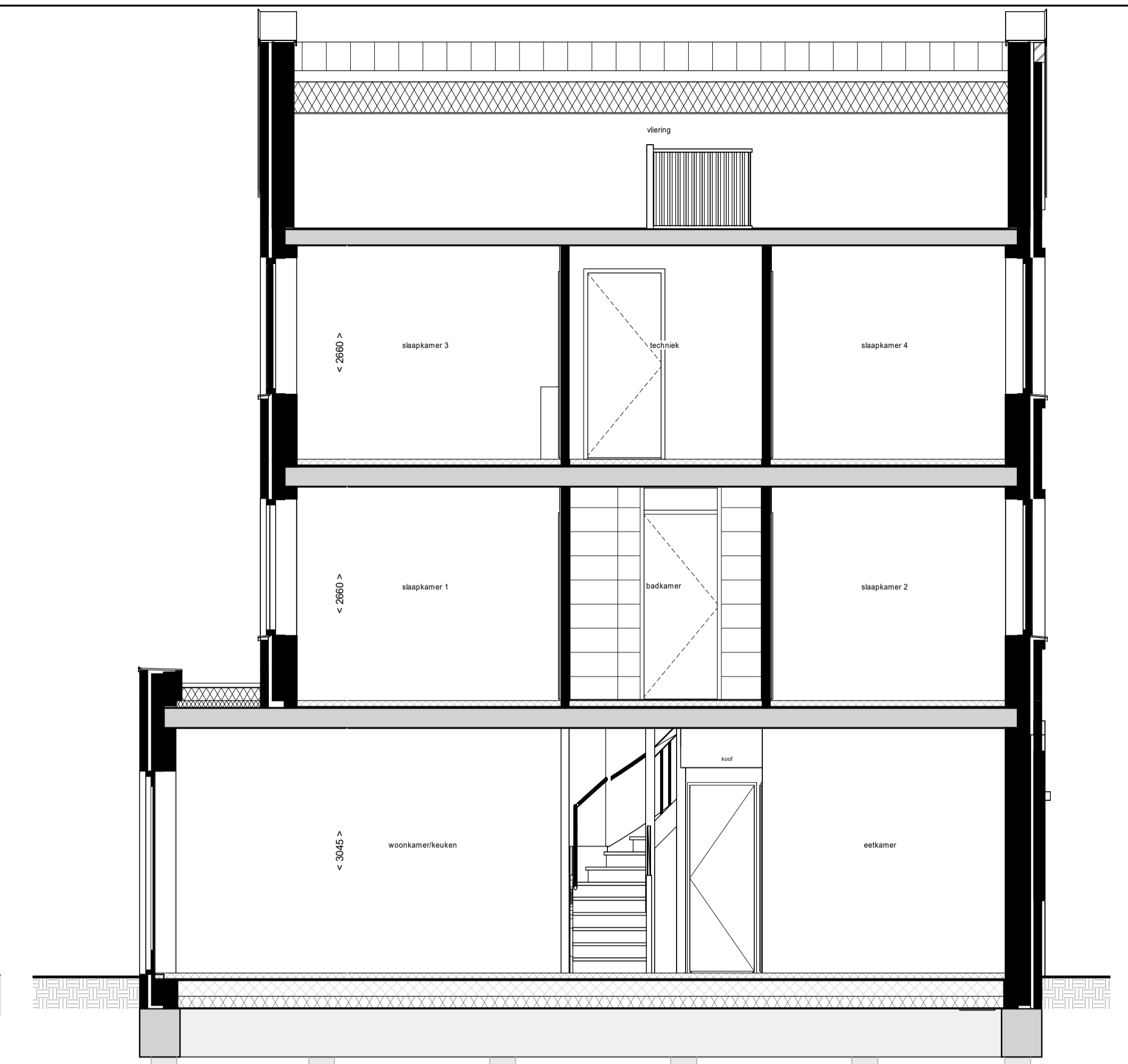
Doorsnede C11
