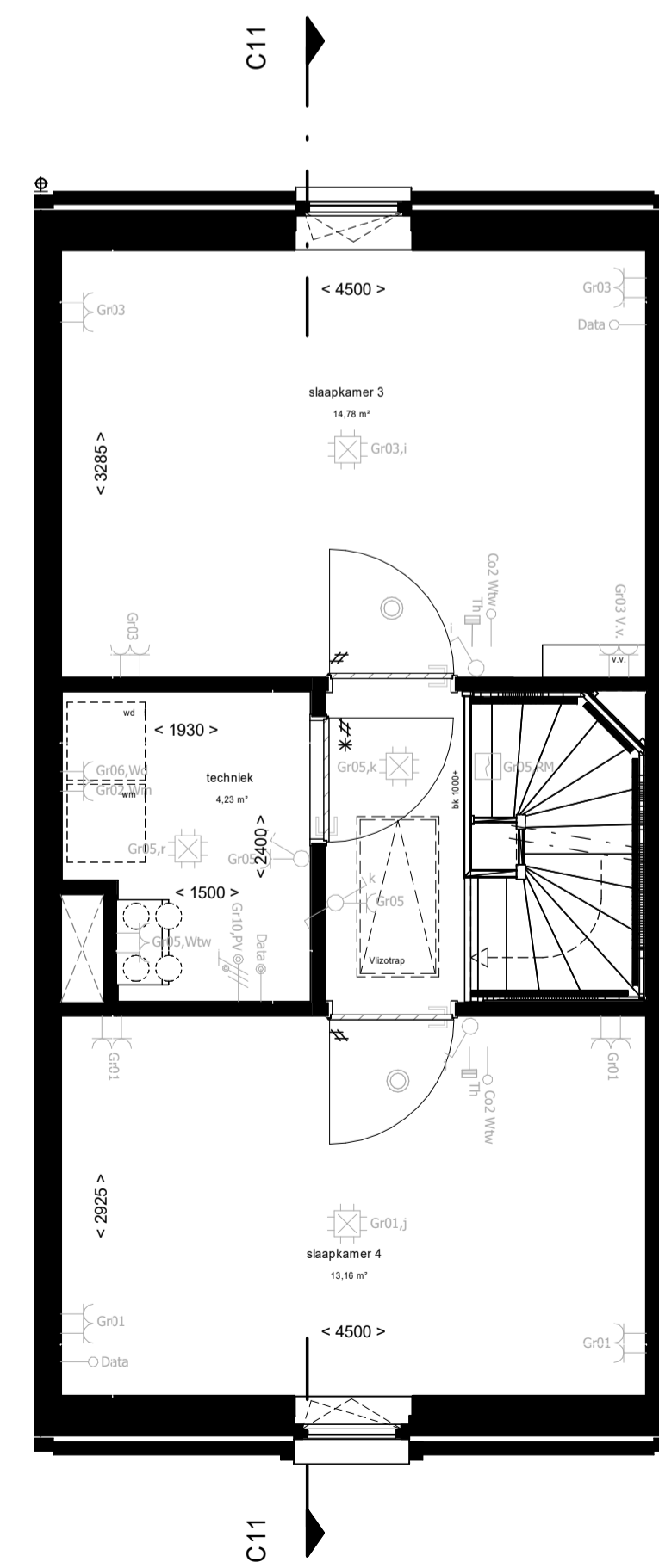
2e verdieping
