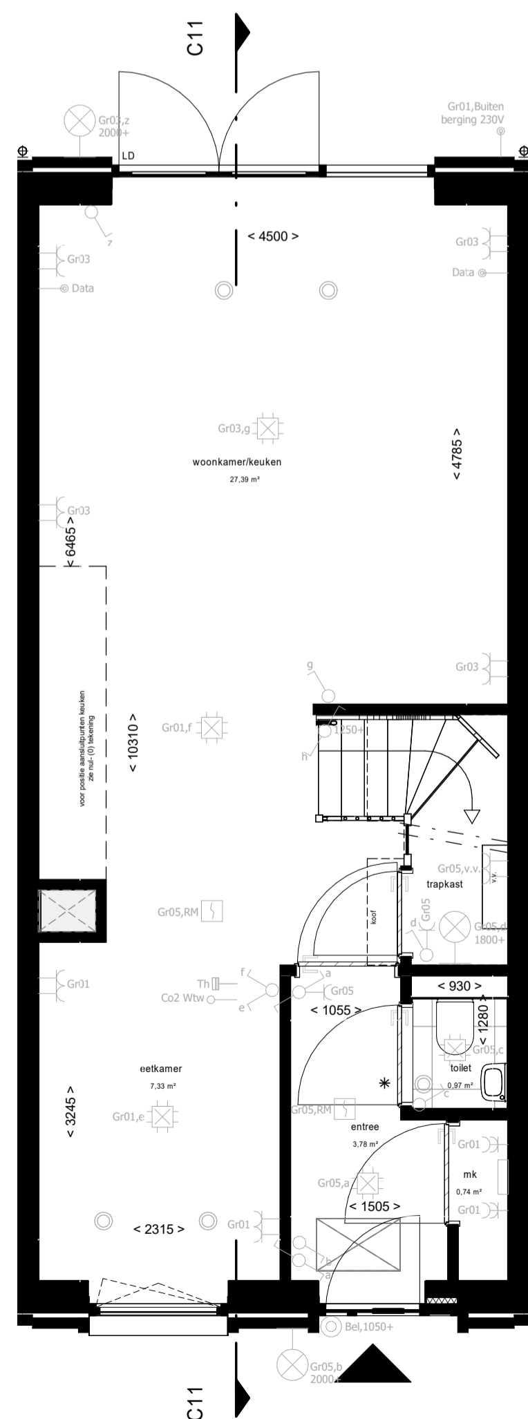
Begane grond
