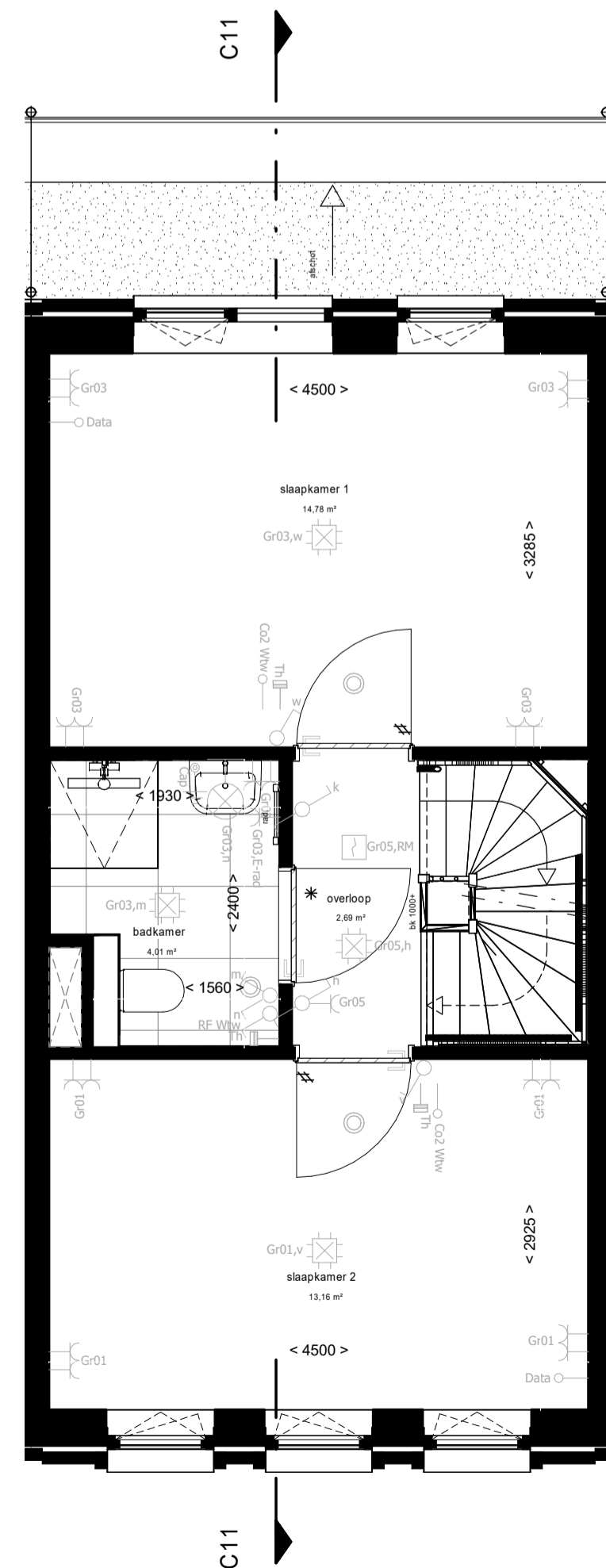
1e verdieping
