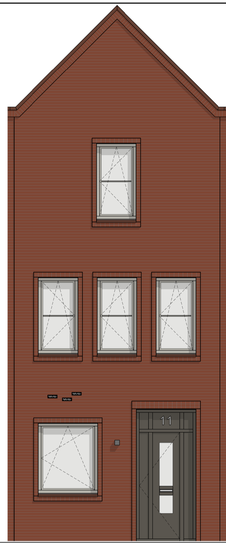
voorgevel
