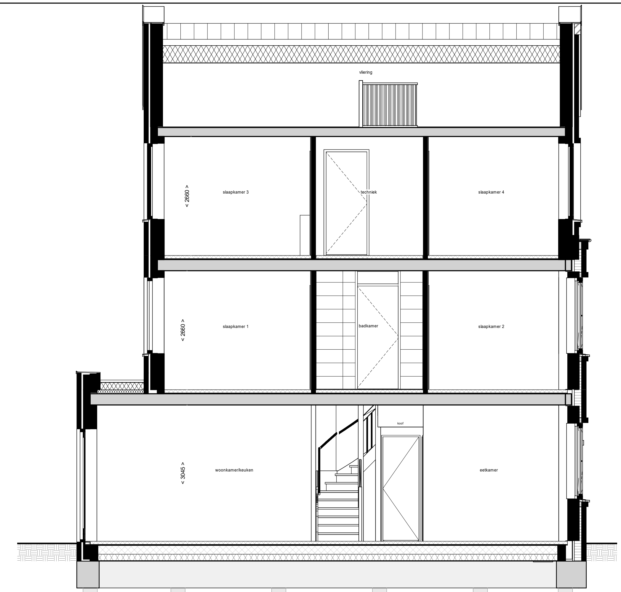
Doorsnede C10
