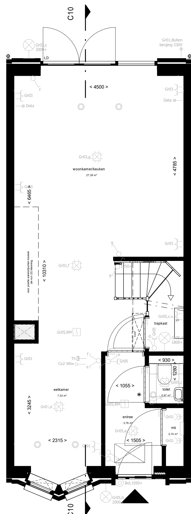
Begane grond
