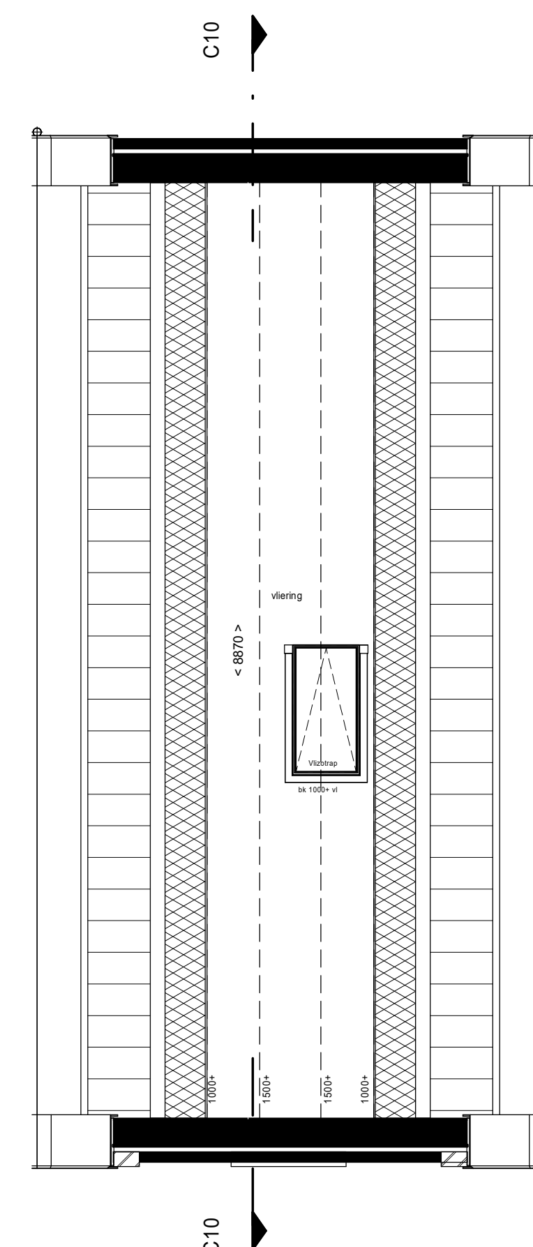
vliering
