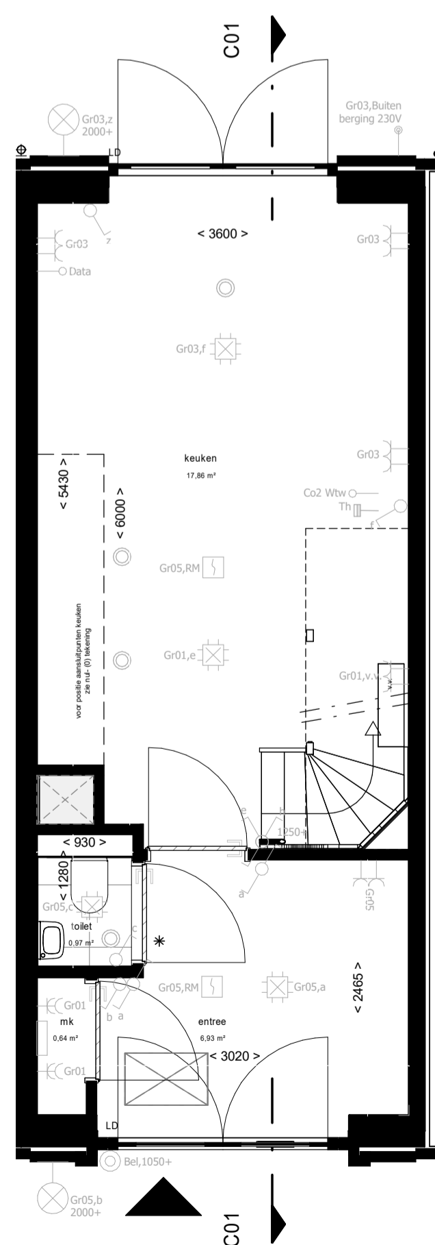
Begane grond
