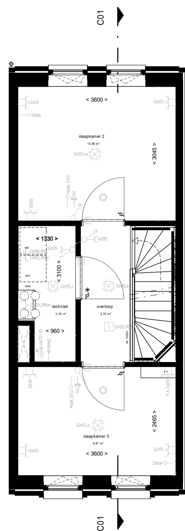
2e verdieping
