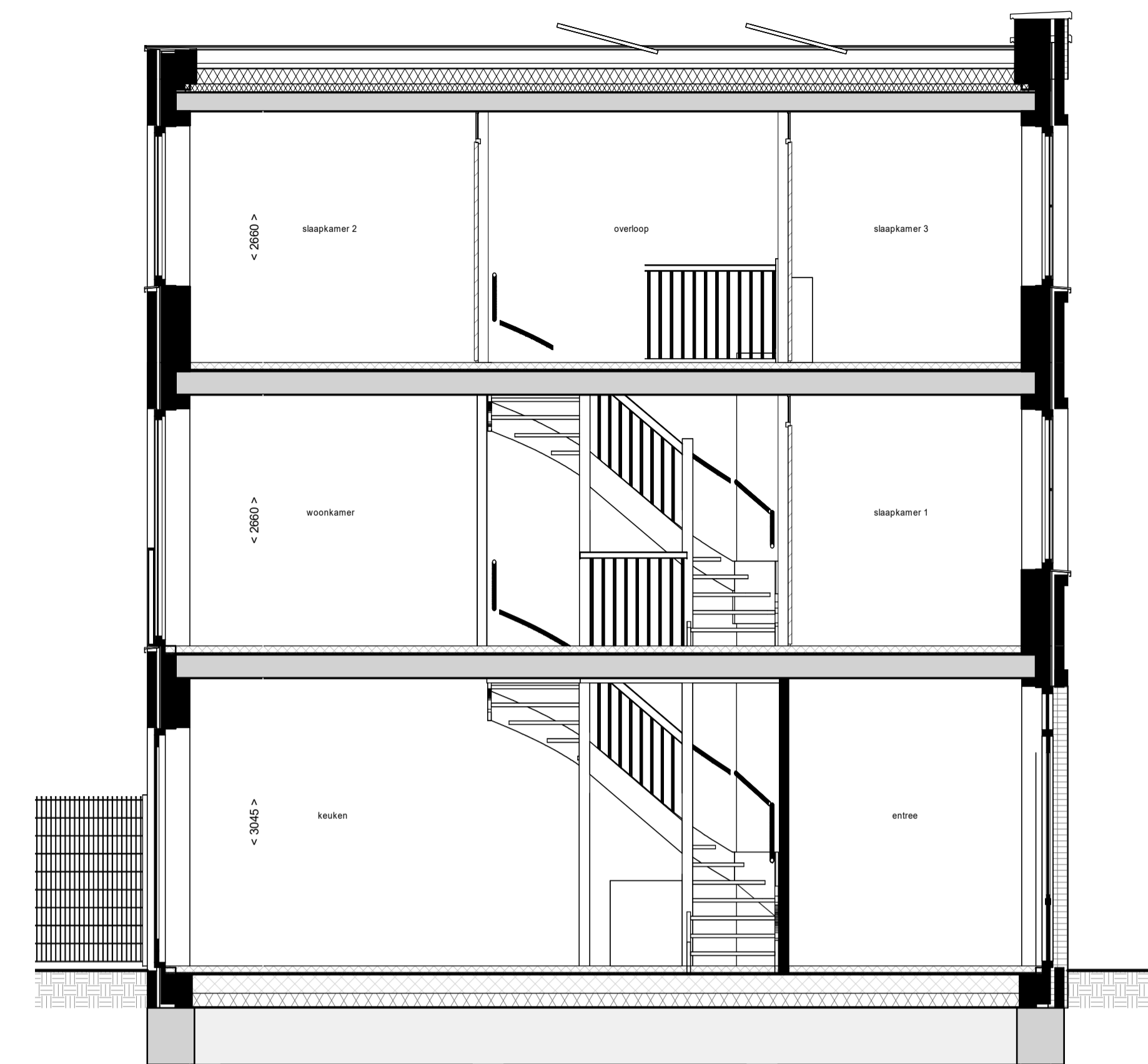
Doorsnede C01
