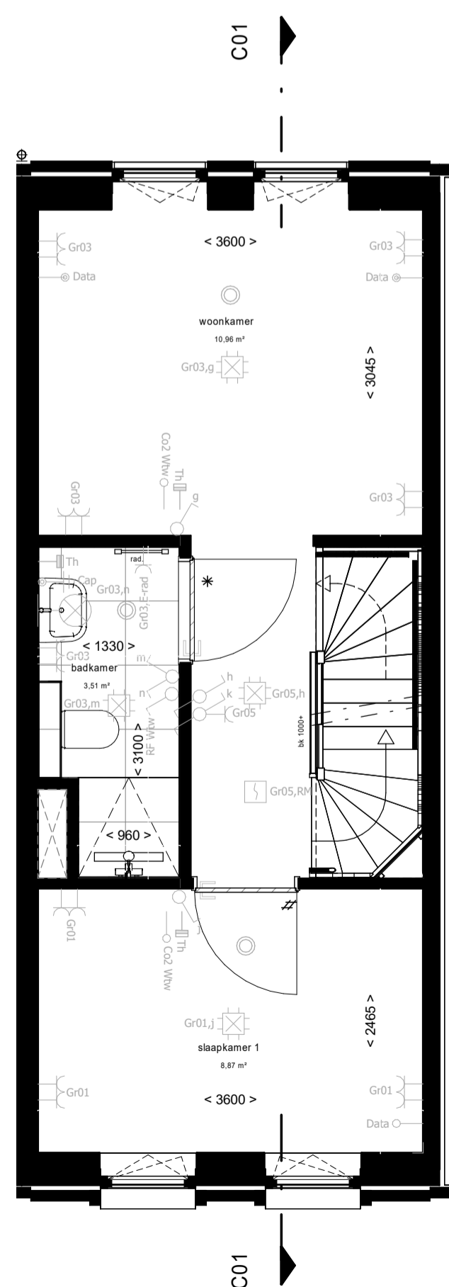
1e verdieping
