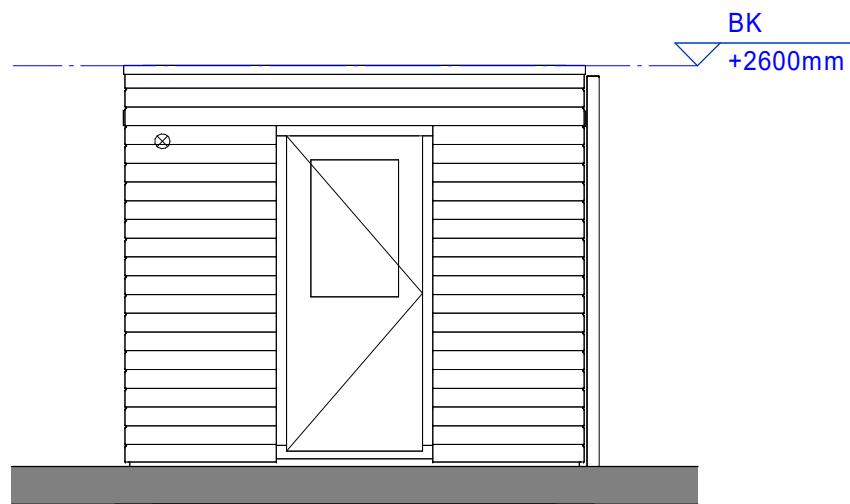
Linker zijaanzicht
