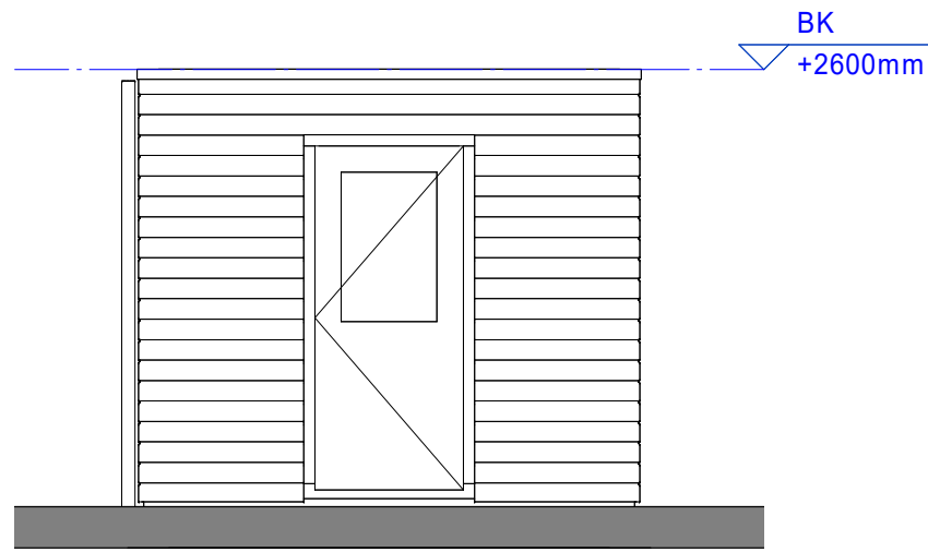
Rechter zijaanzicht
