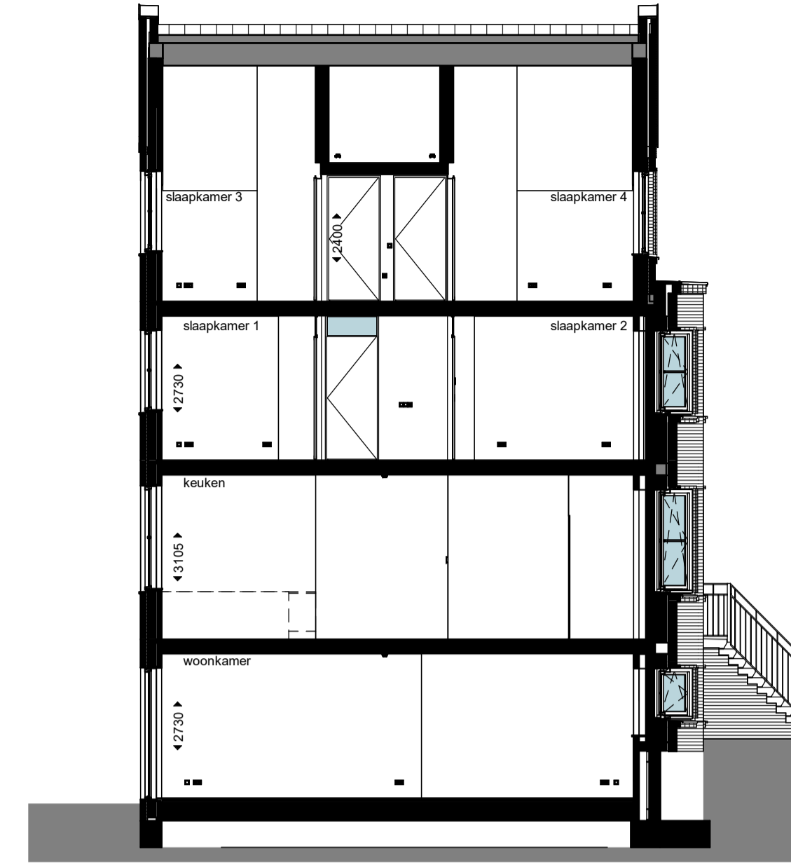
doorsnede
