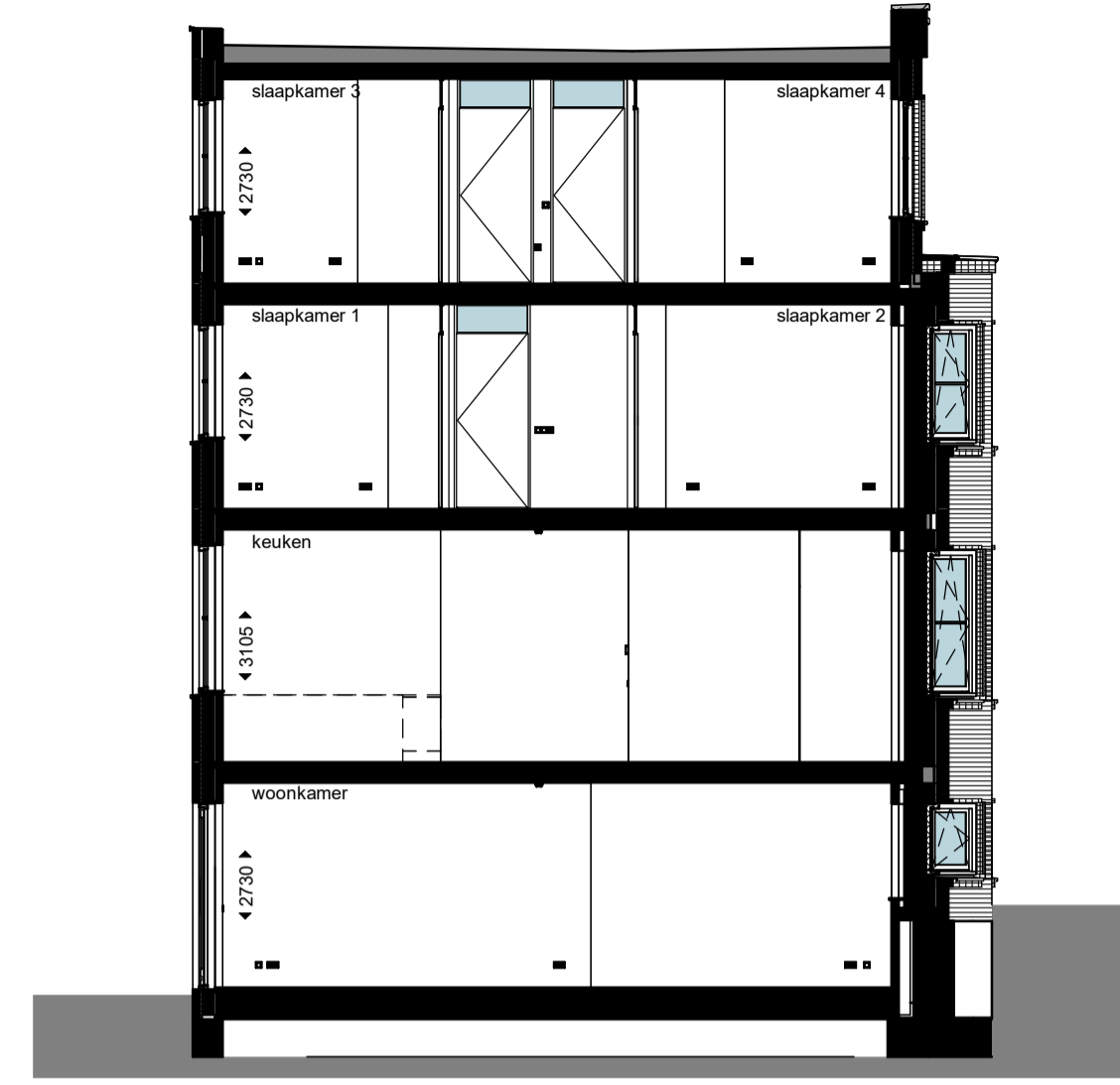
doorsnede
