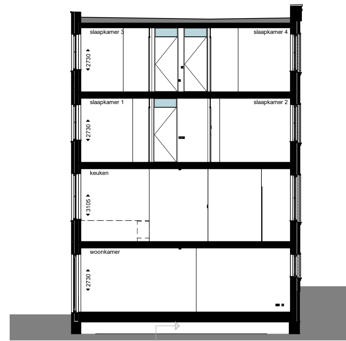
doorsnede
