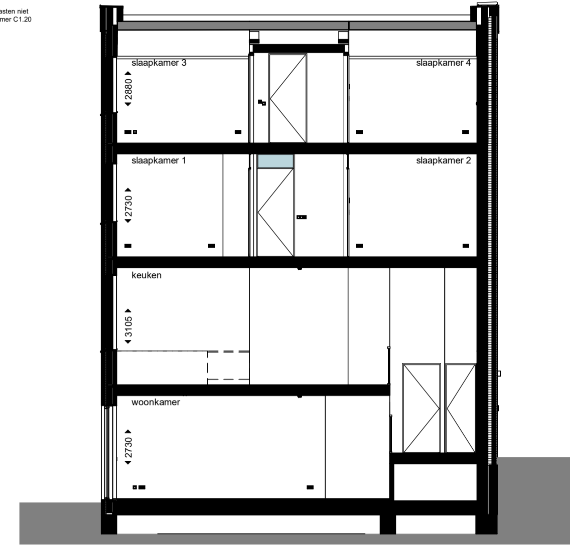
doorsnede
