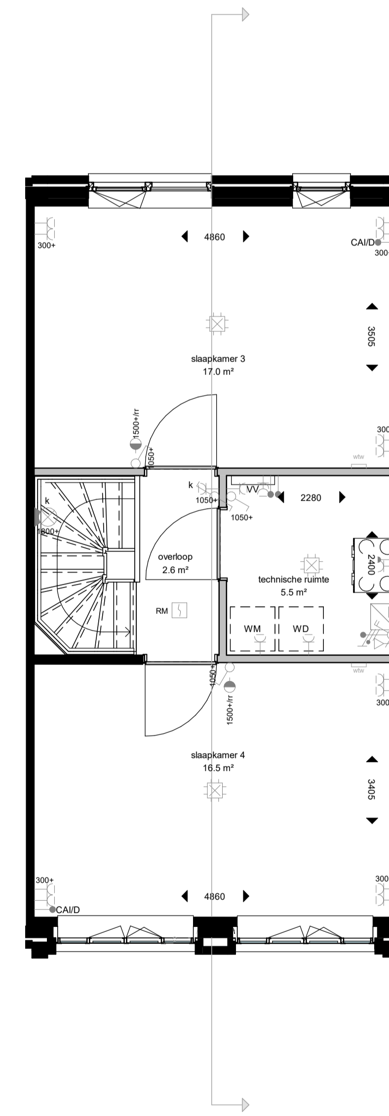
tweede verdieping
