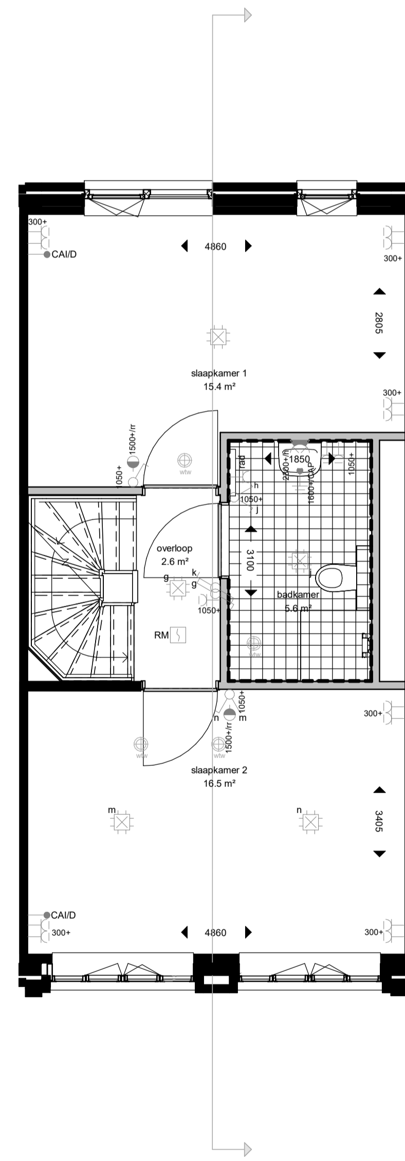
eerste verdieping
