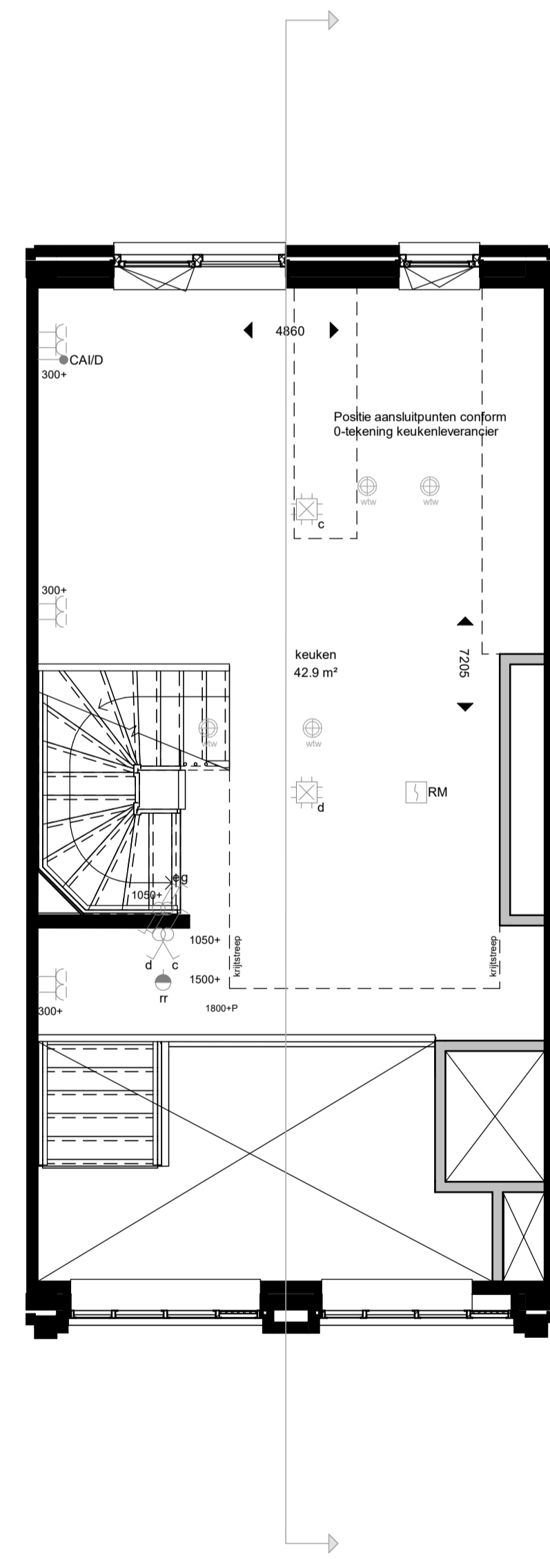
begane grond
