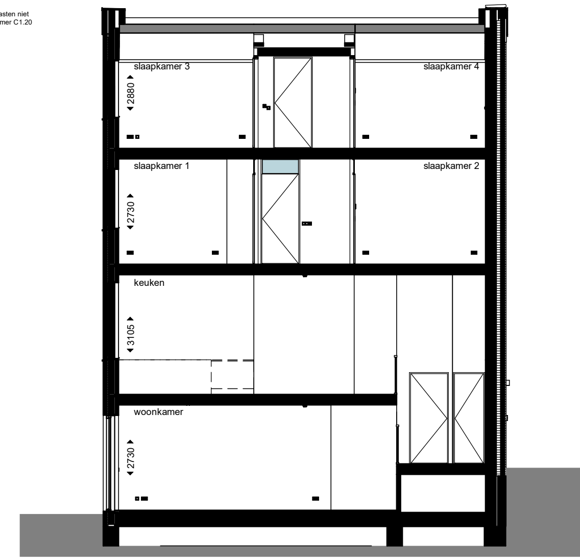
doorsnede
