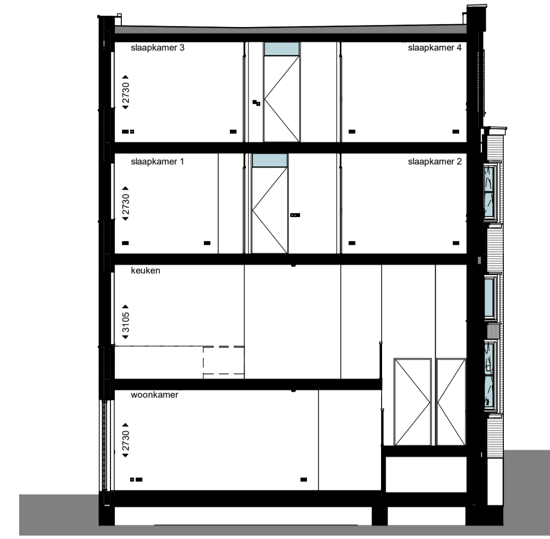
doorsnede
