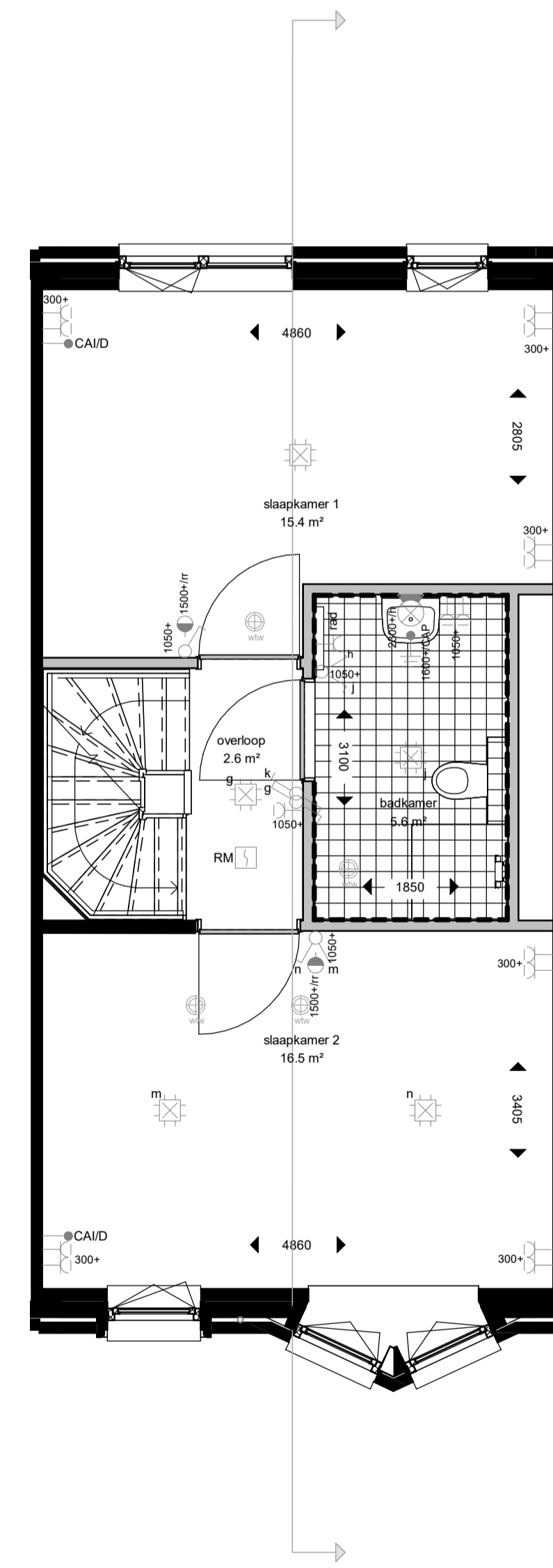
eerste verdieping
