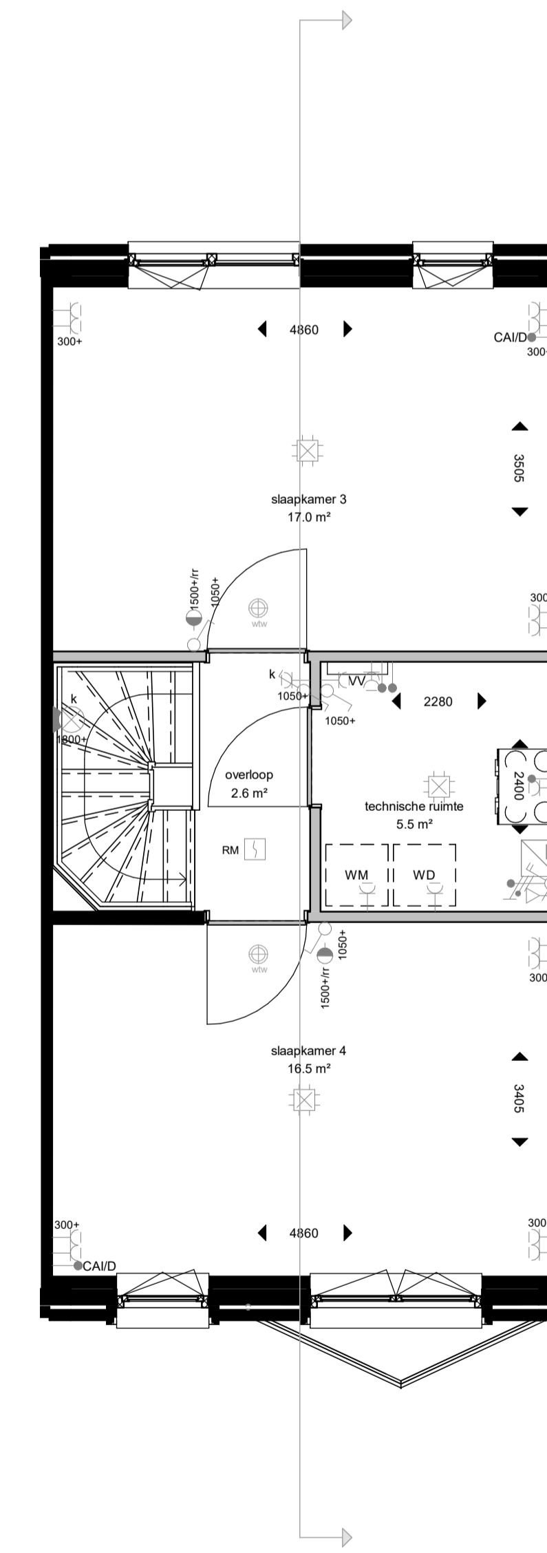
tweede verdieping
