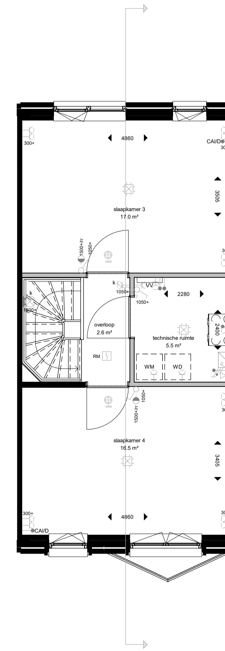
tweede verdieping
