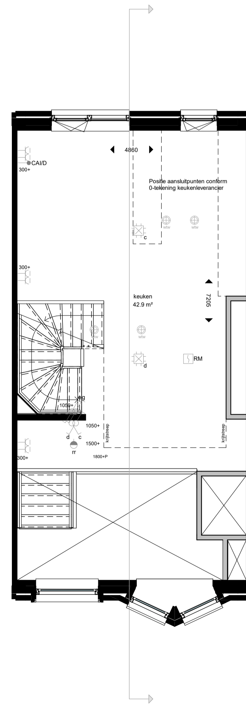
begane grond
