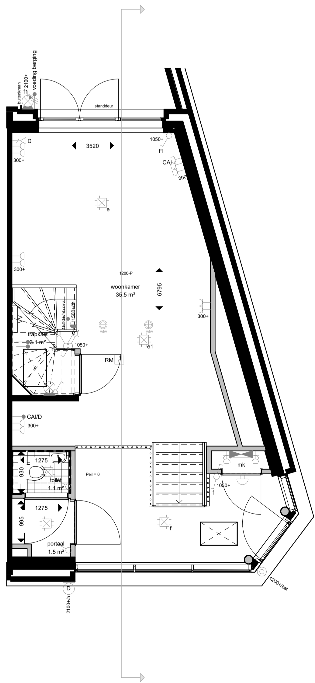
souterrain
