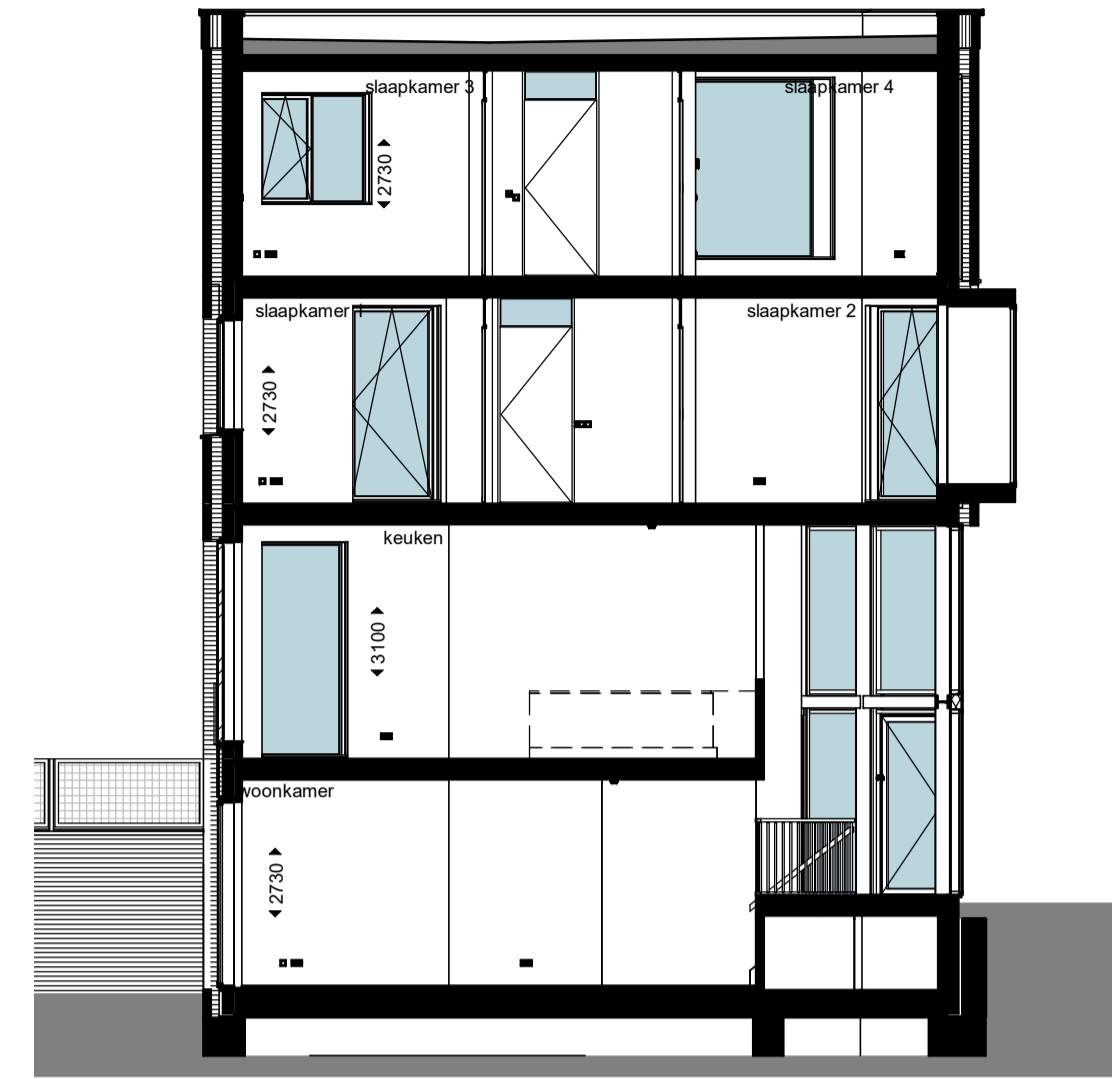
doorsnede
