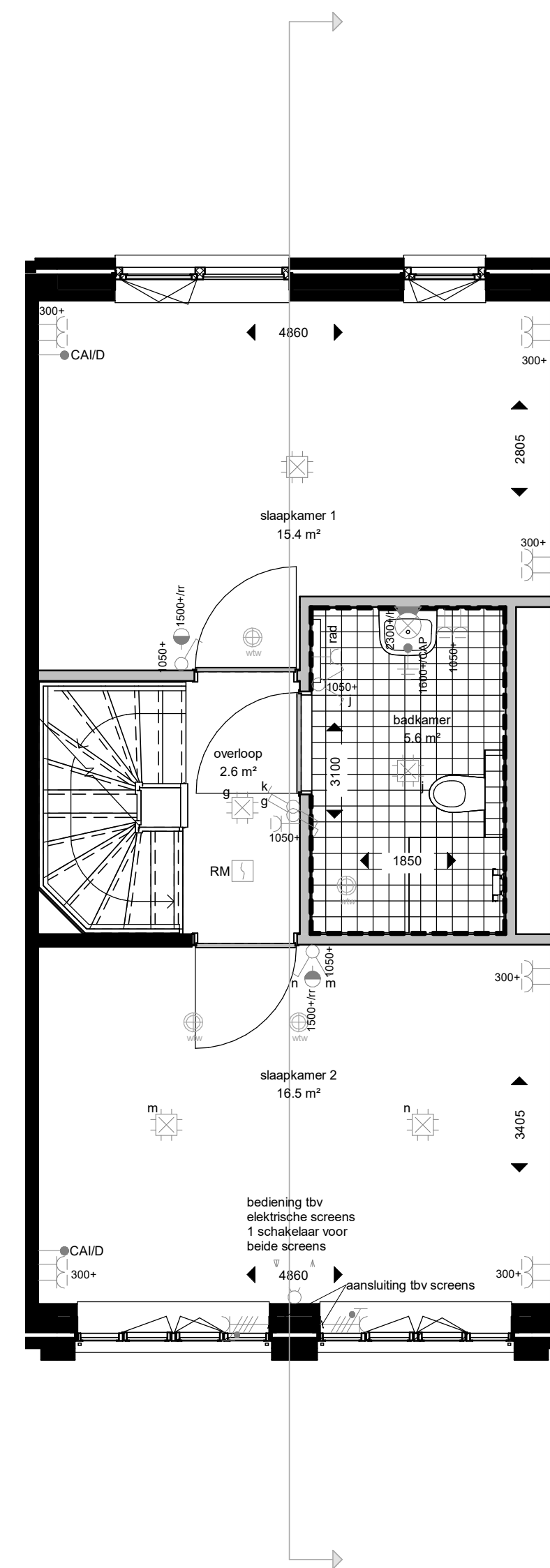
eerste verdieping
