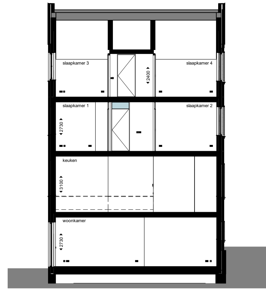
doorsnede
