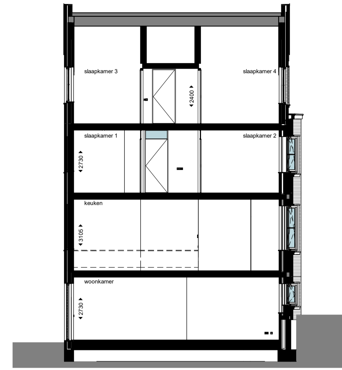
doorsnede
